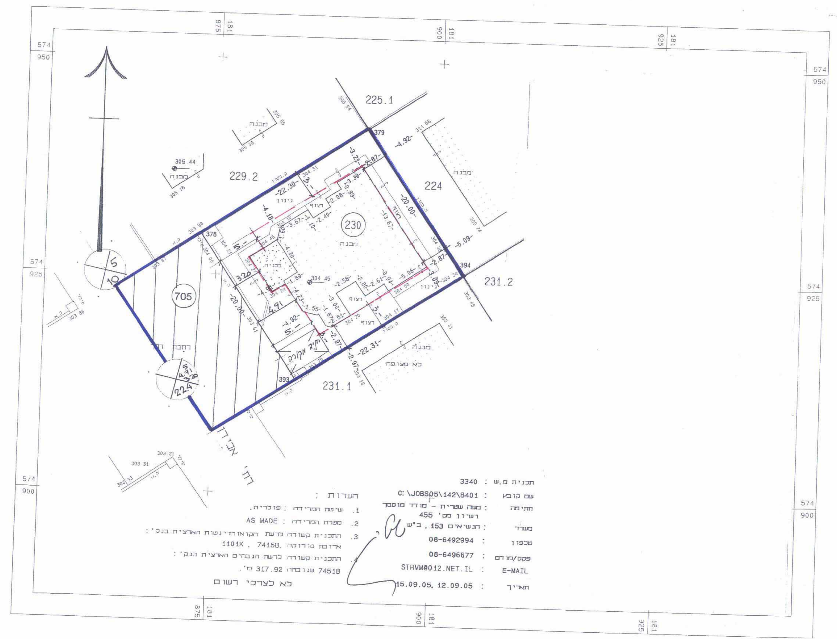
מצב מוצע 1:250
