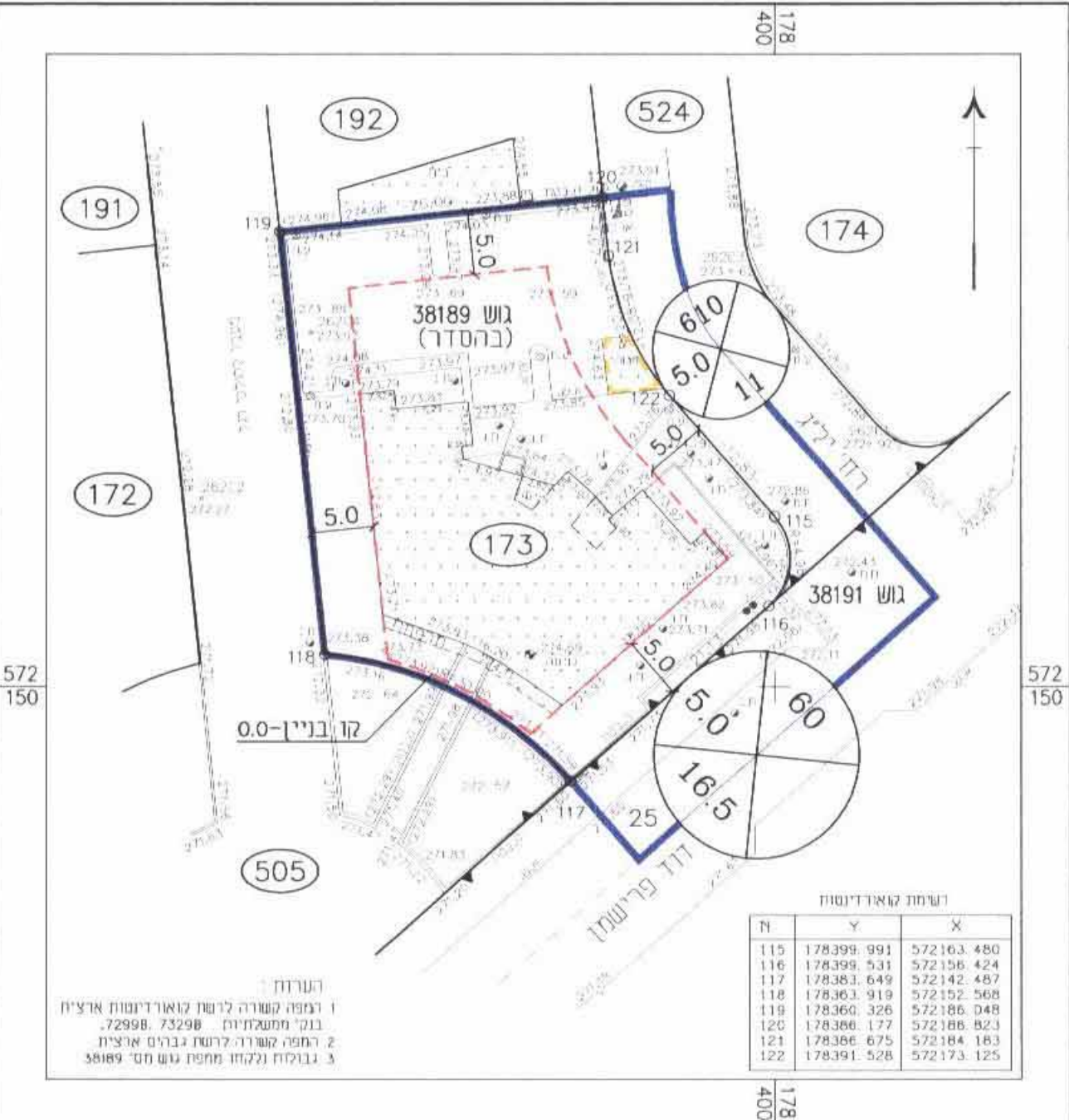
מצב קיים ומוצע 1:500
