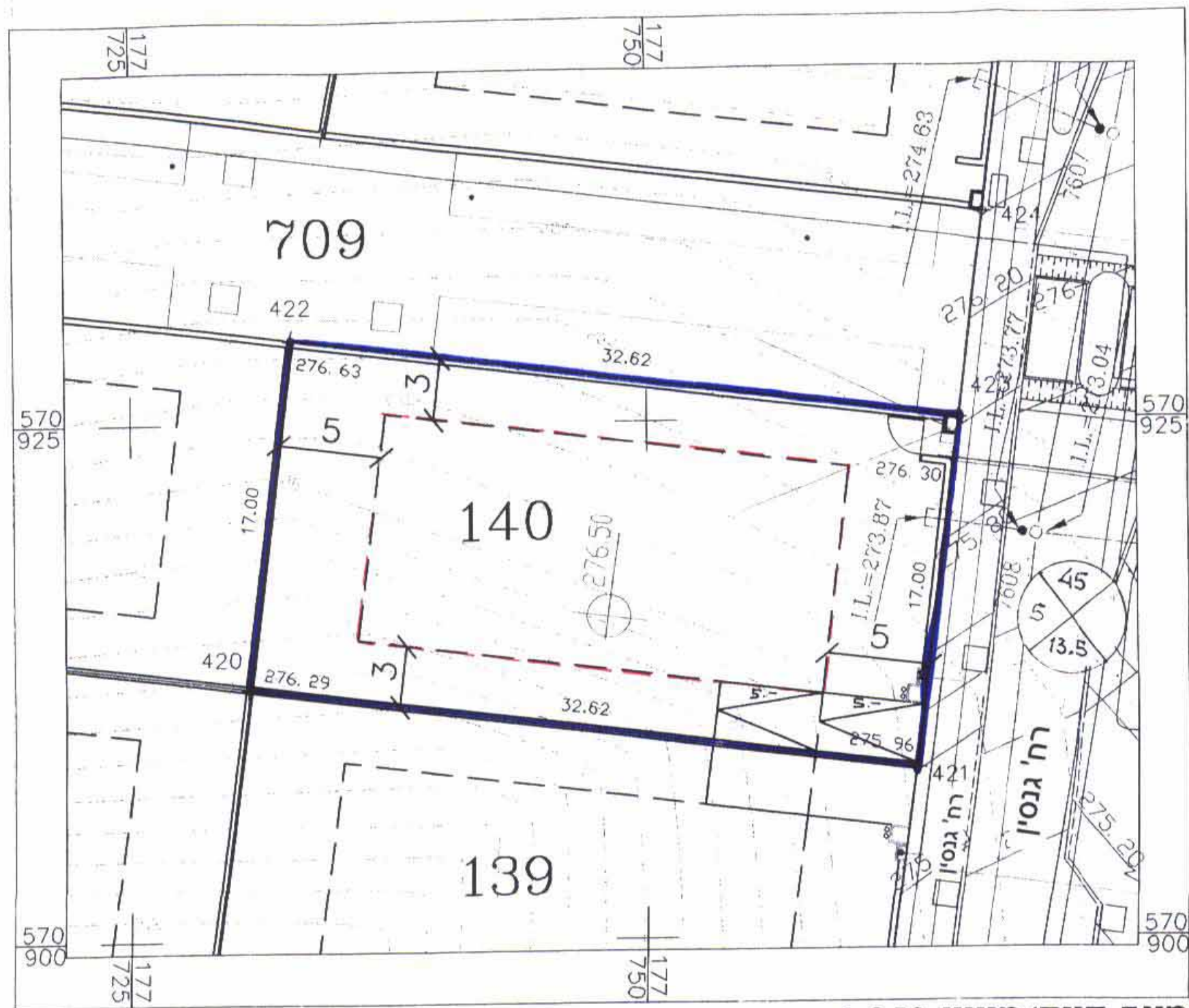
מצב קיים/מוצע 1:250
