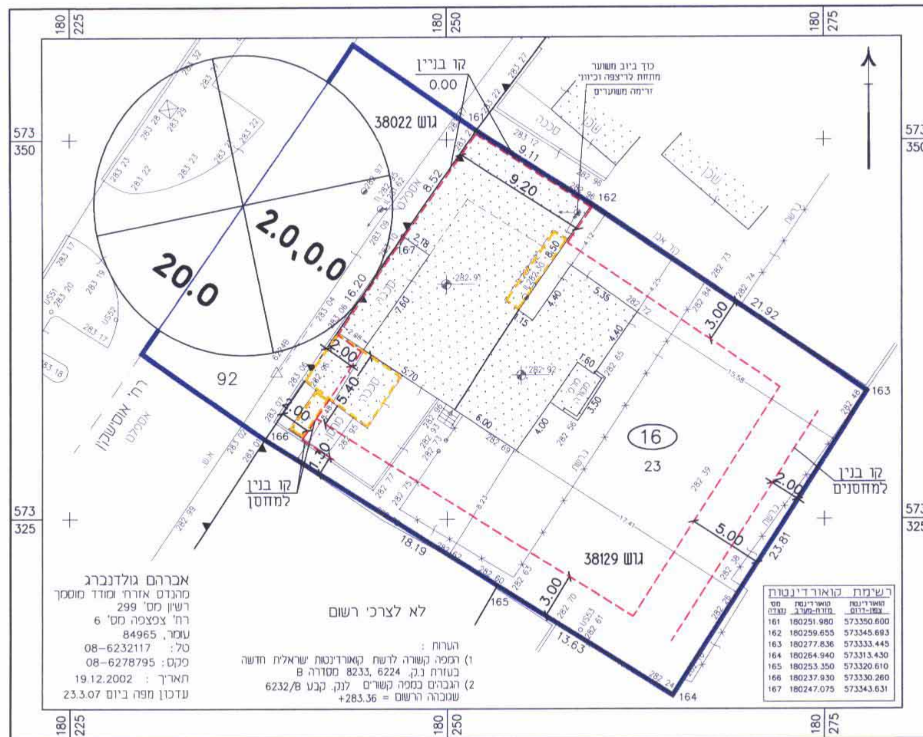
מצב מוצע 1:250
