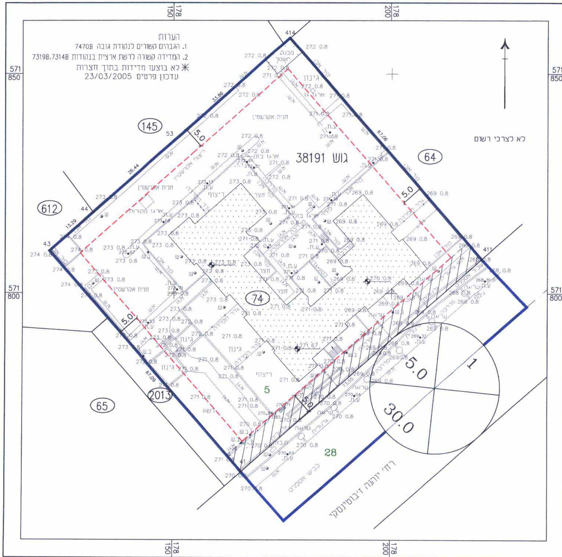
מצב קיים ומוצע 1:500
