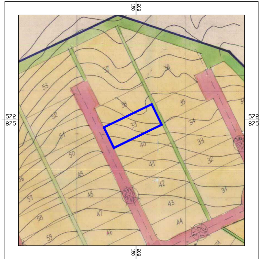
תרשים סביבה מצב מאושר לפי תכנית 337\03\7 1:1500 קני"מ
