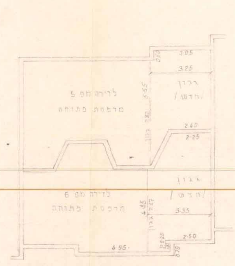
מרפסת גג קנה מדה: 1 : 100
