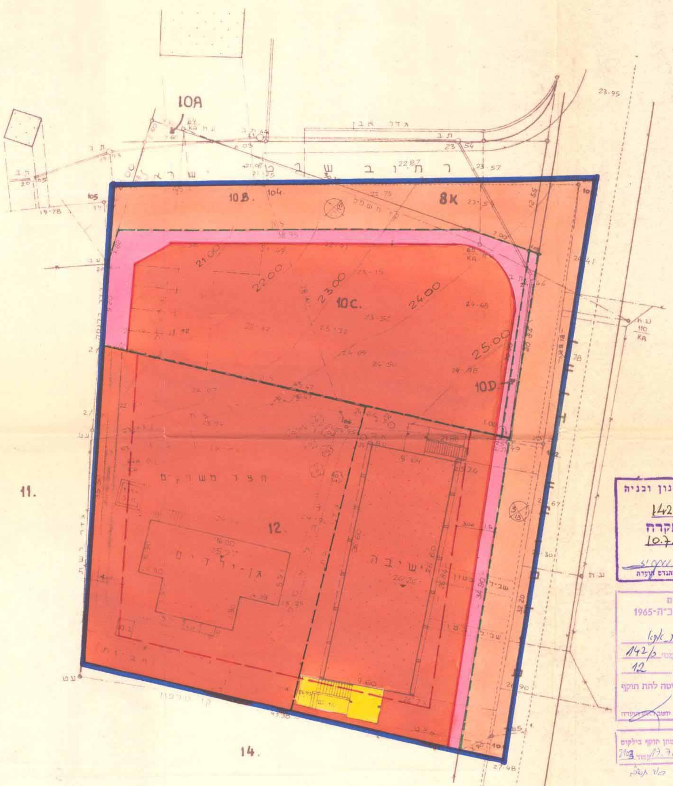
תרשים המקום 1:5000
