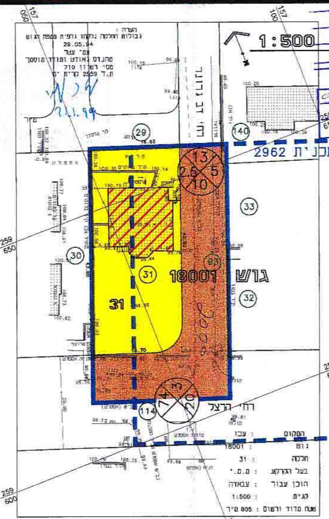
תכנית 2962 קיים 1:500
