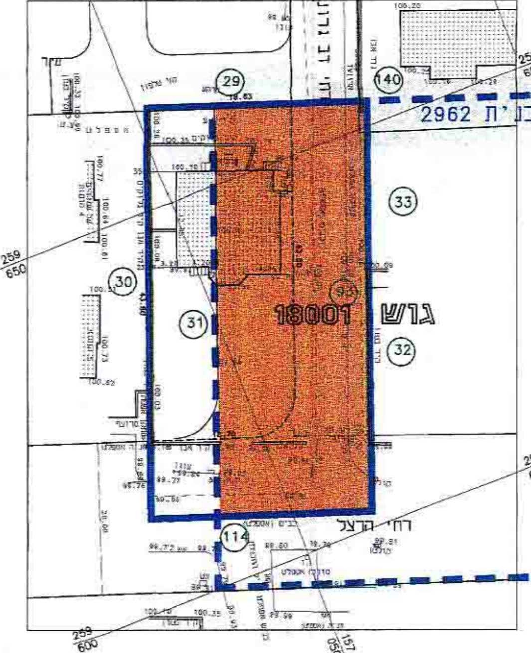
תכנית 2962 קיים 1:500
