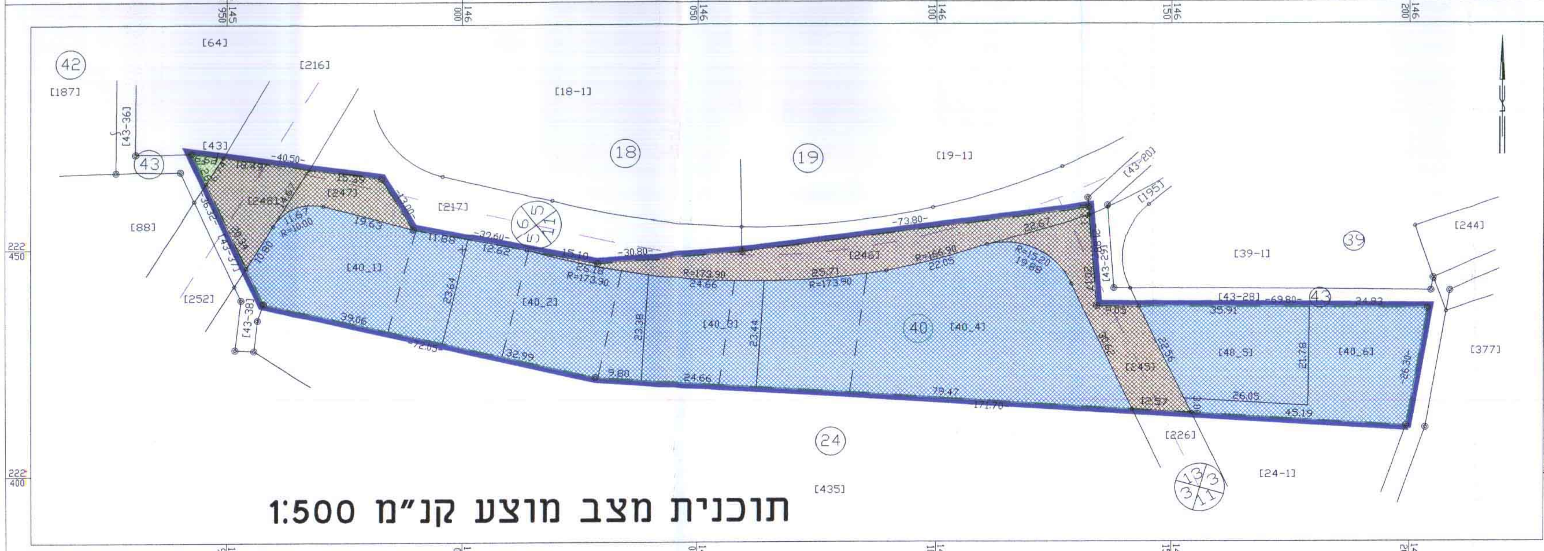
תוכנית מצב קיים קנ"מ 1:500
