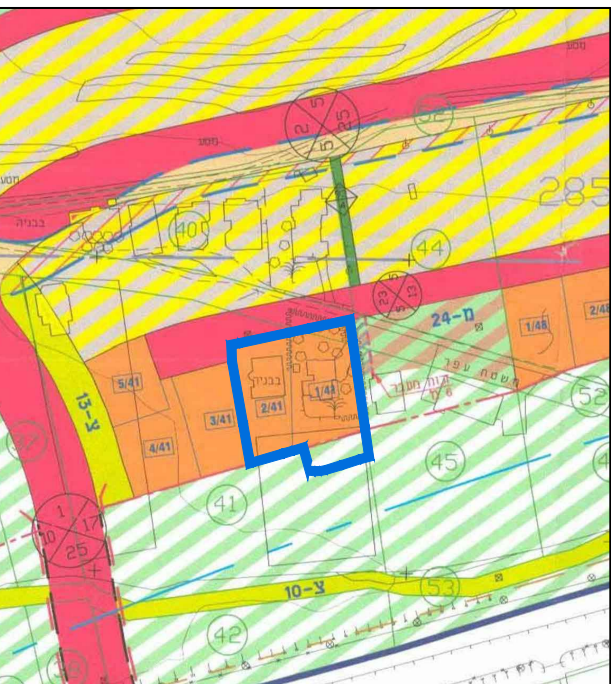
תרשים סביבה קנימ 1:2500
