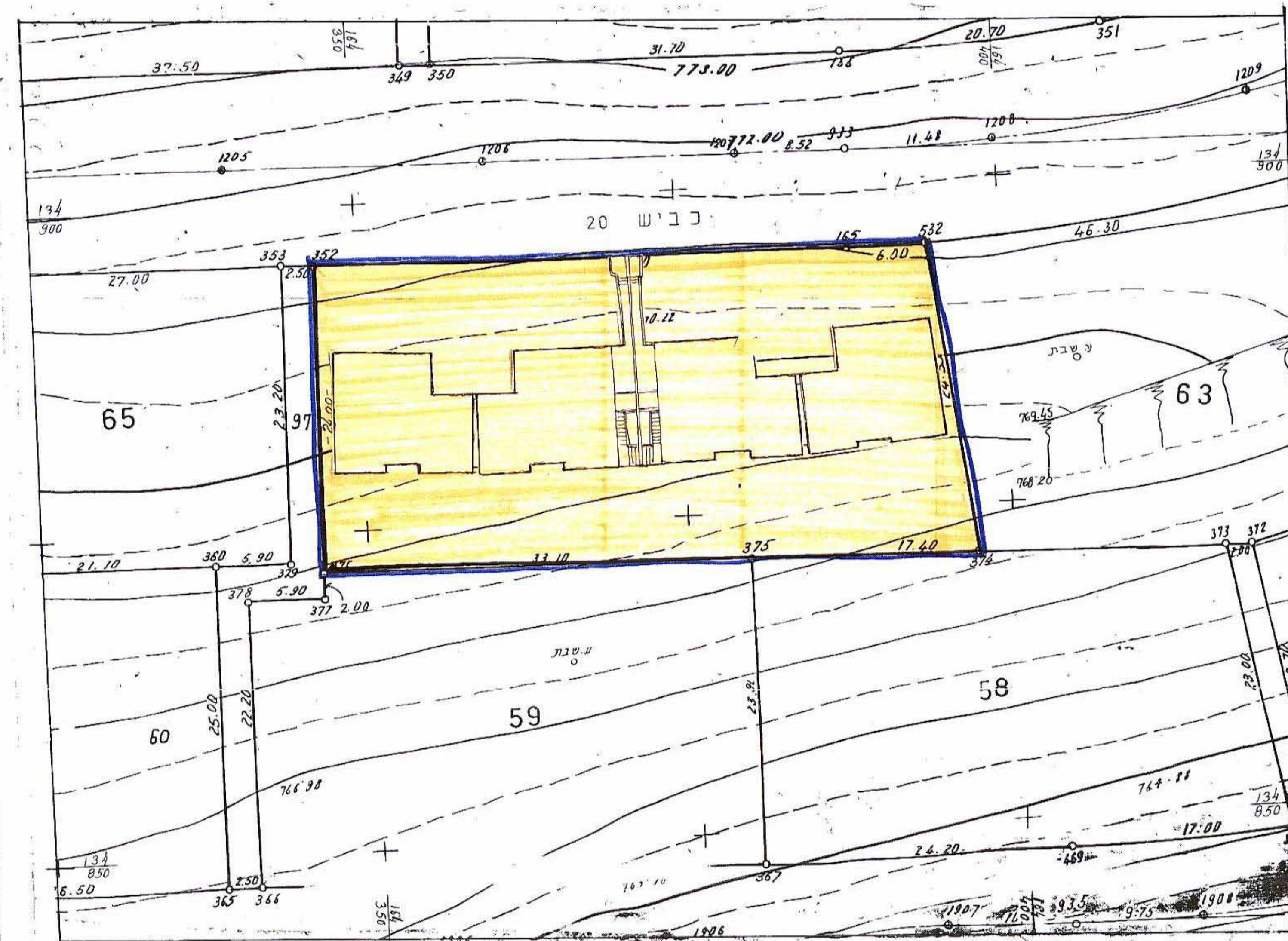
מפה טופוגרפית קנה 1:250
