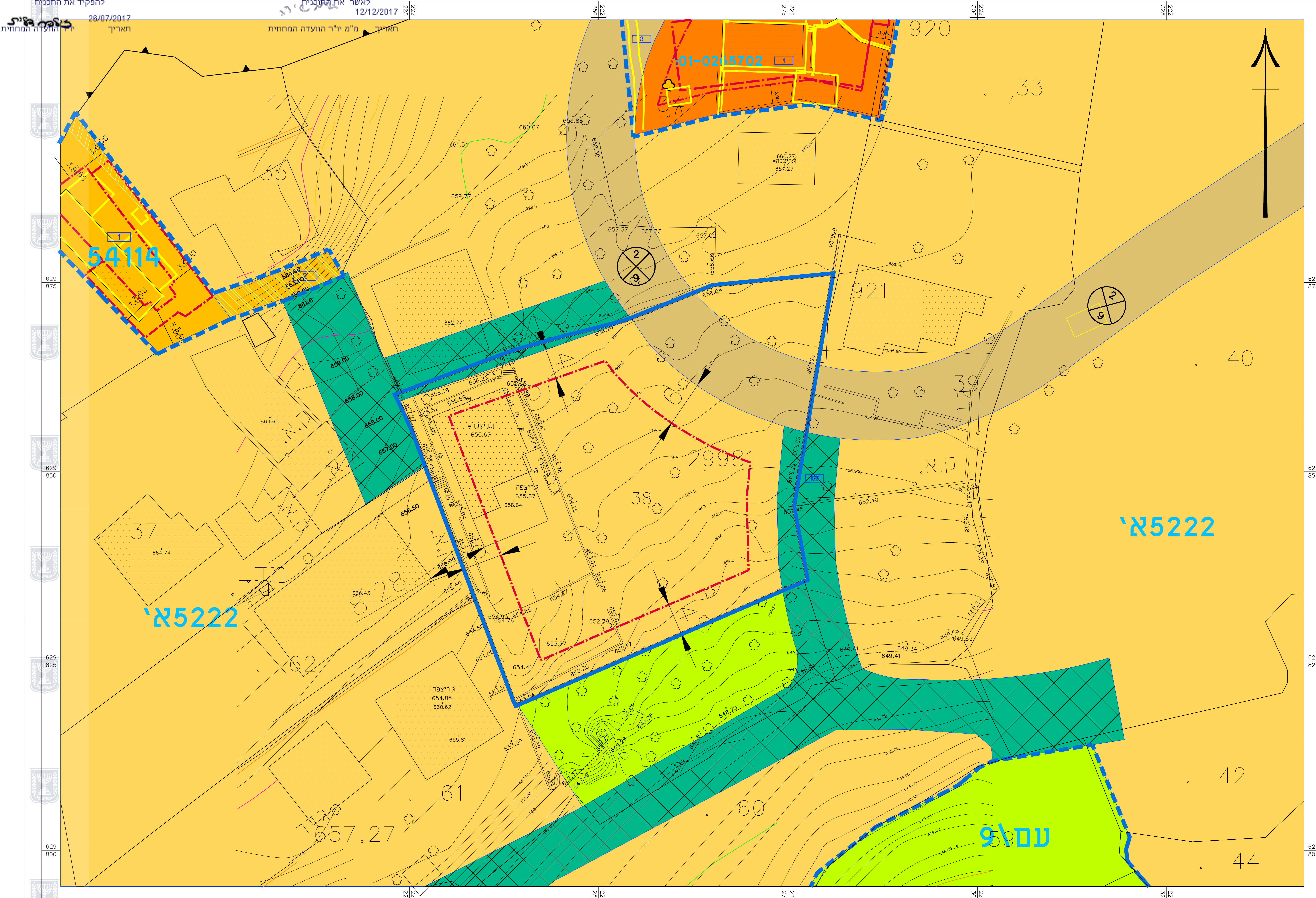
מצב מאושר ע"פי תכנית 5222א', 9\54114, 0265702-101 קני"מ 1:250
