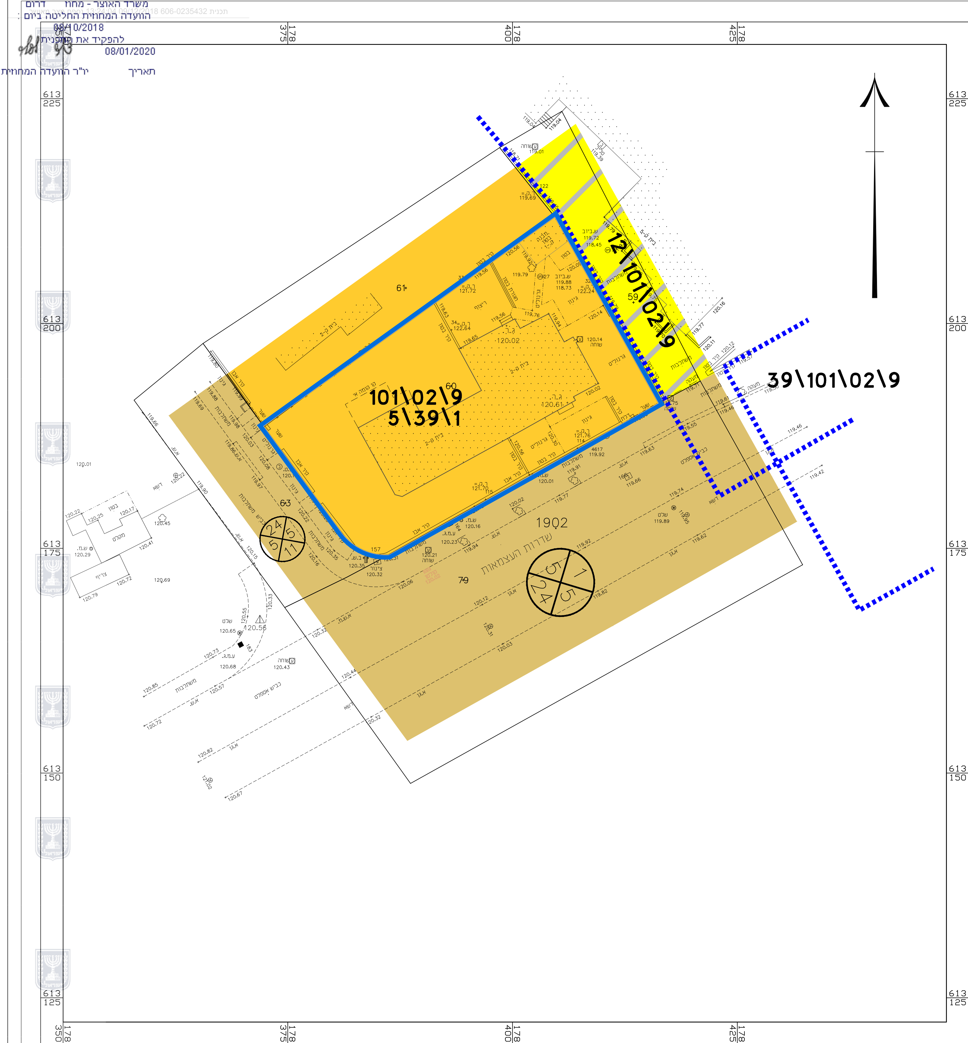
מצב מאושר קנ"מ 1 : 250
