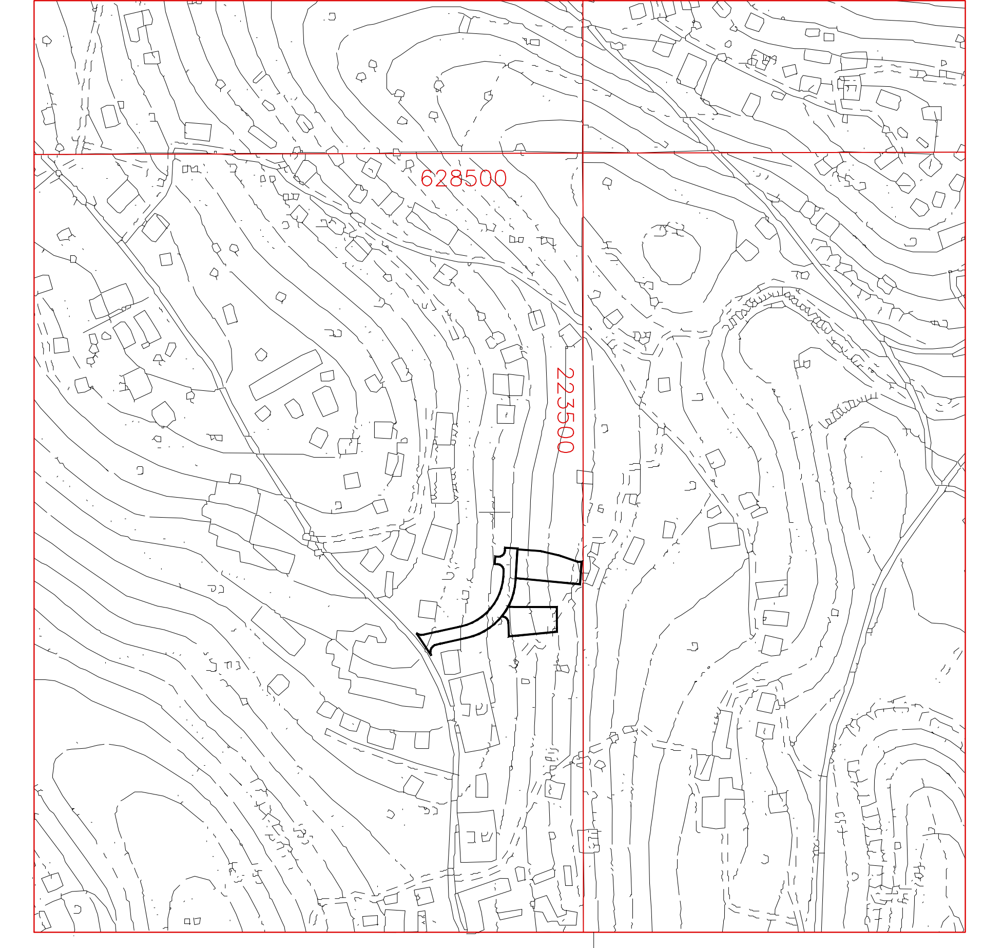
תרשים הסביבה קנה מידה 1:5000
