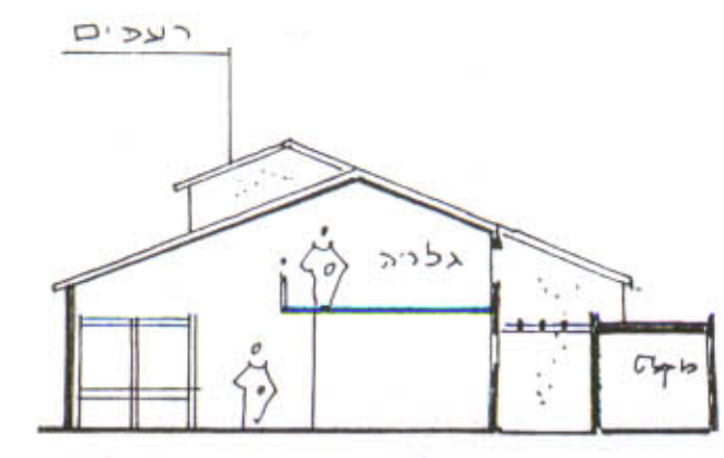
חתך א-א 1:200
