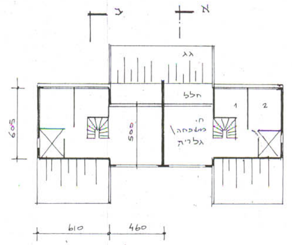
תכנית קומה א' 1:200
