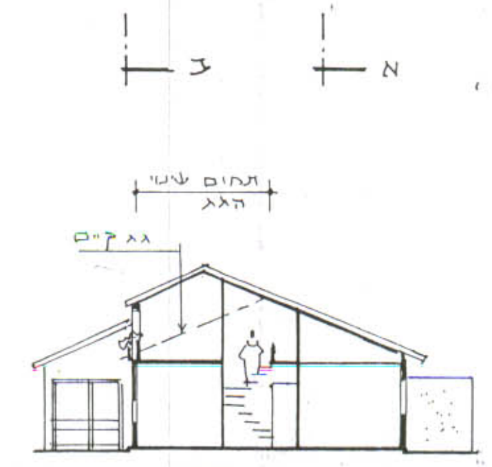
חתך ב-ב 1:200
