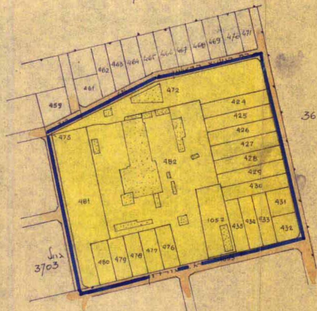
מצב קיים 1:2500
