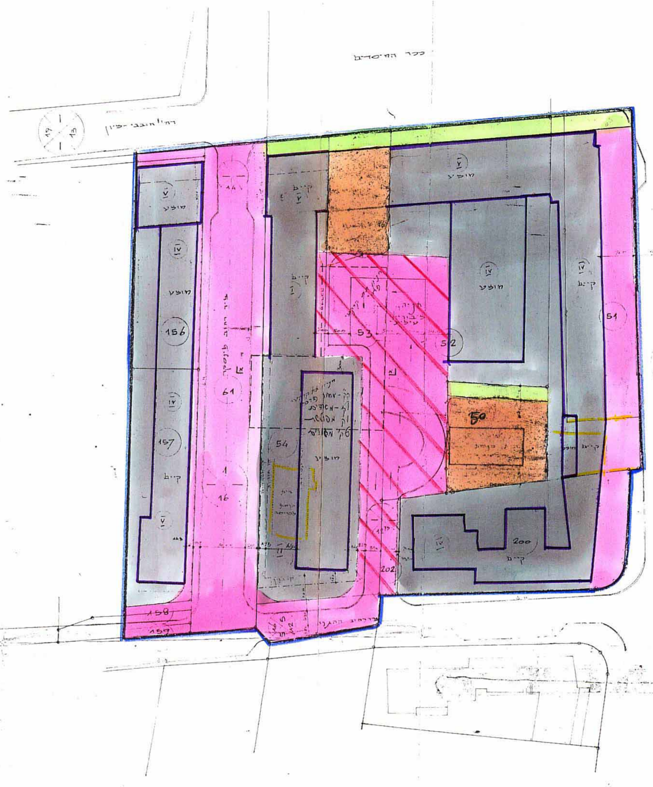
תרשים המגרש 1:500
