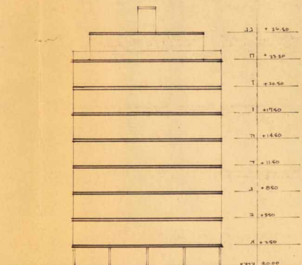
חתך 1:250
