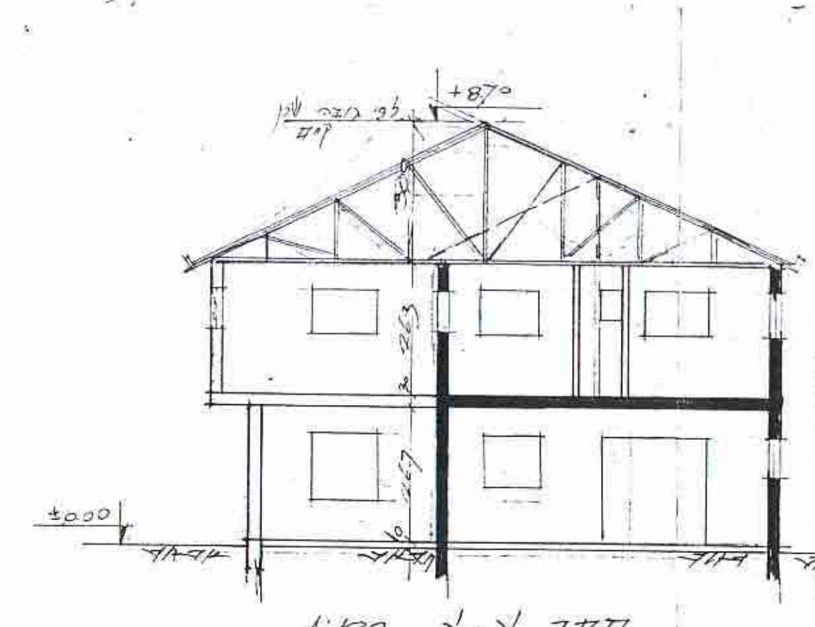
חזית מזרחית 1:100
