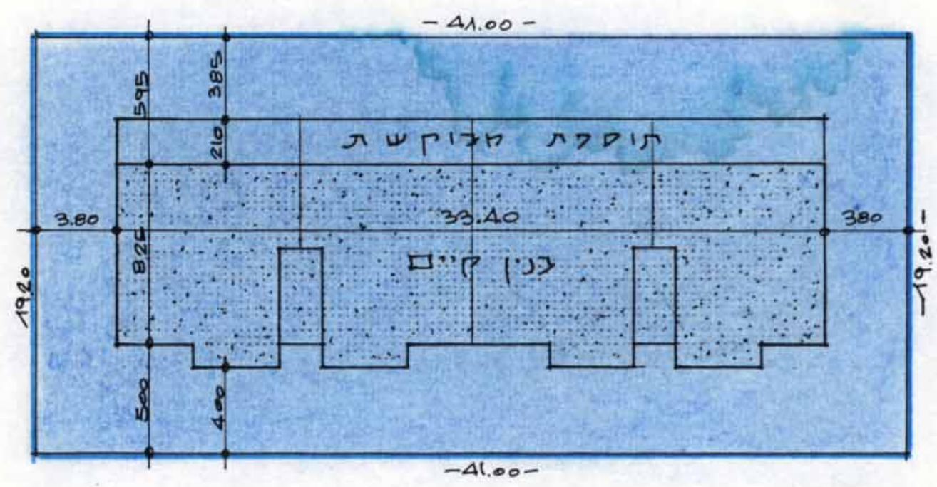
● תרשים המגרש 11/250
