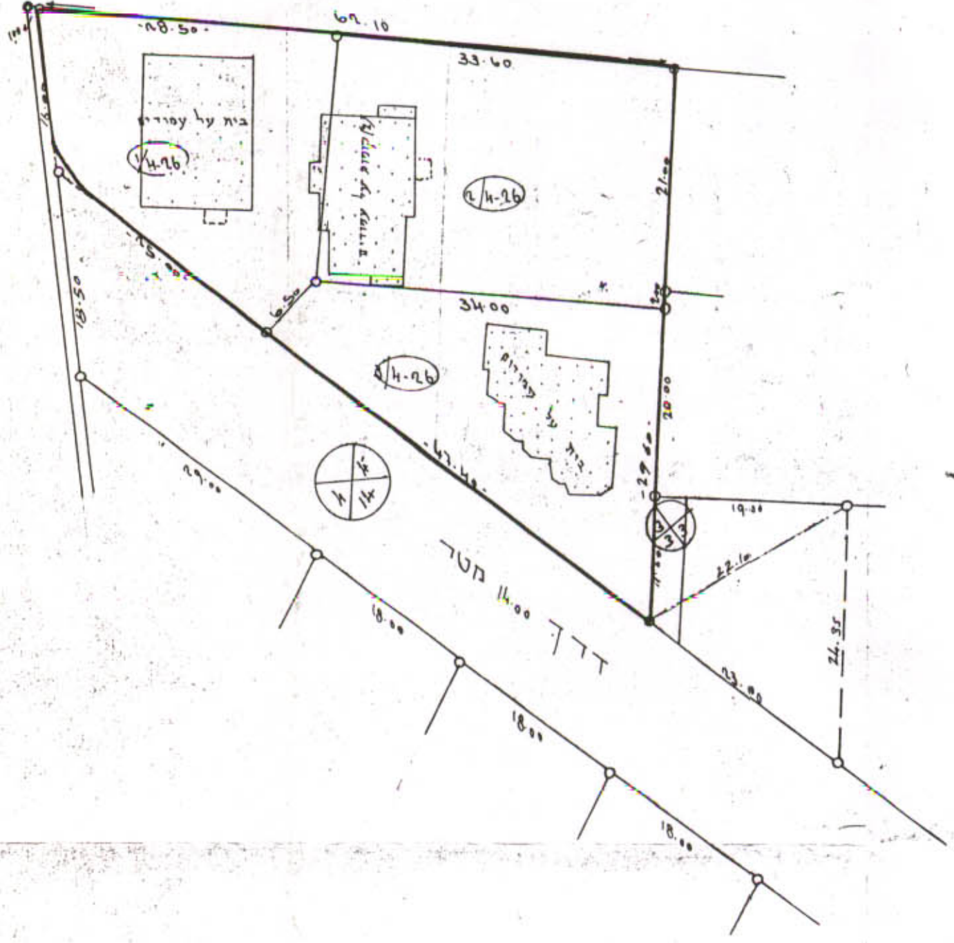
תרשיב המצב הקיים קנה 1:500 לשר חמ' 839
