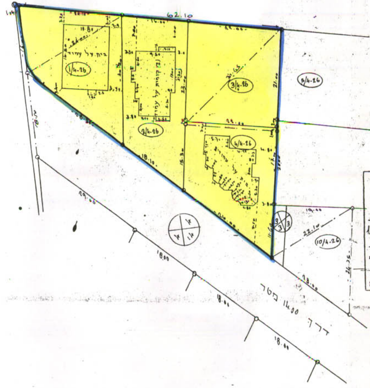
תרשיב המצב המוצע קנה 1:500
