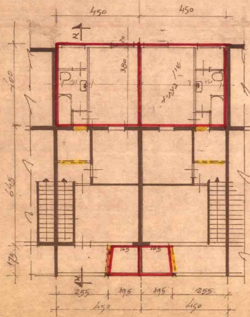
תכנית קומה א 1:100
