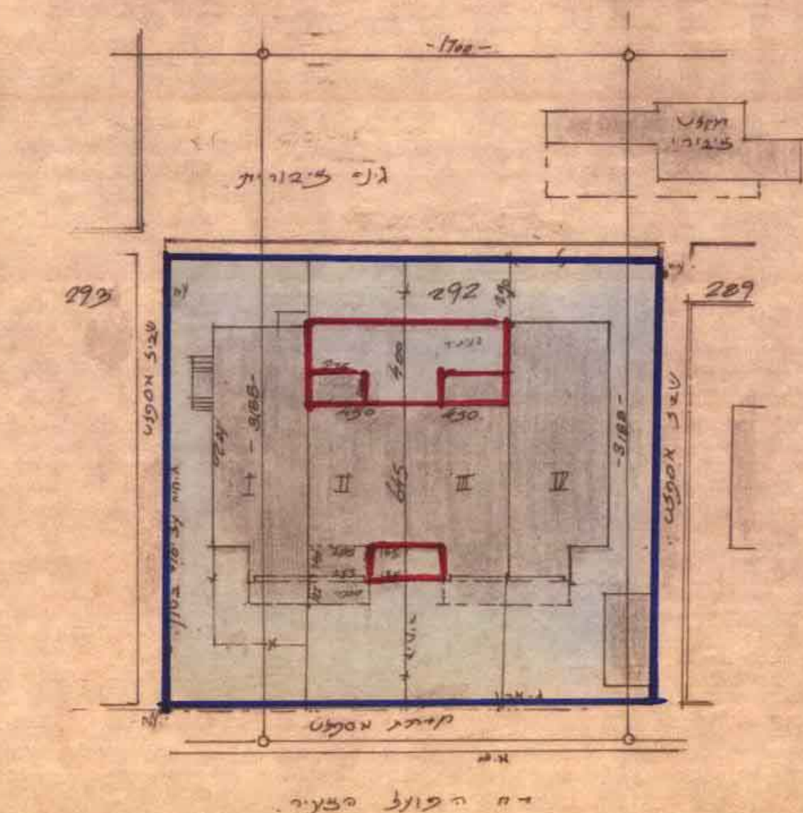
דרישיון מפרט 1:250 מ 25 ב מו"מ
