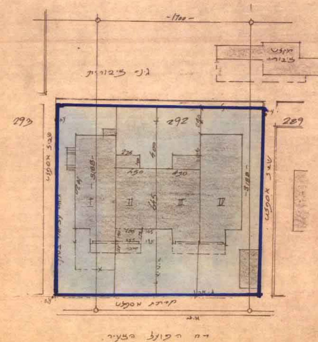
דרישיון מפרט 1:250 מ 25 קו"מ
