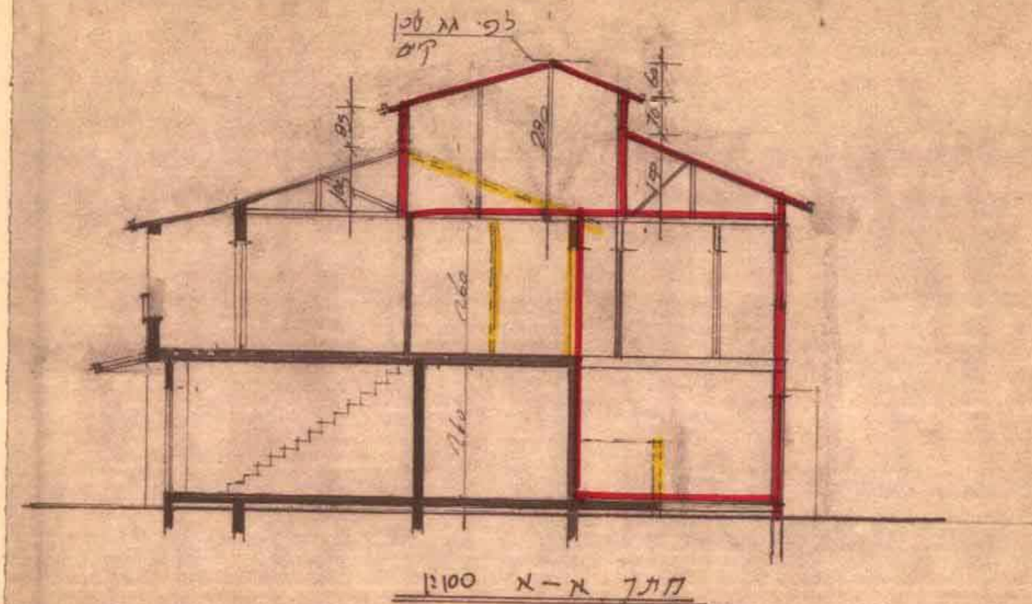
חיתך א-א 1:100
