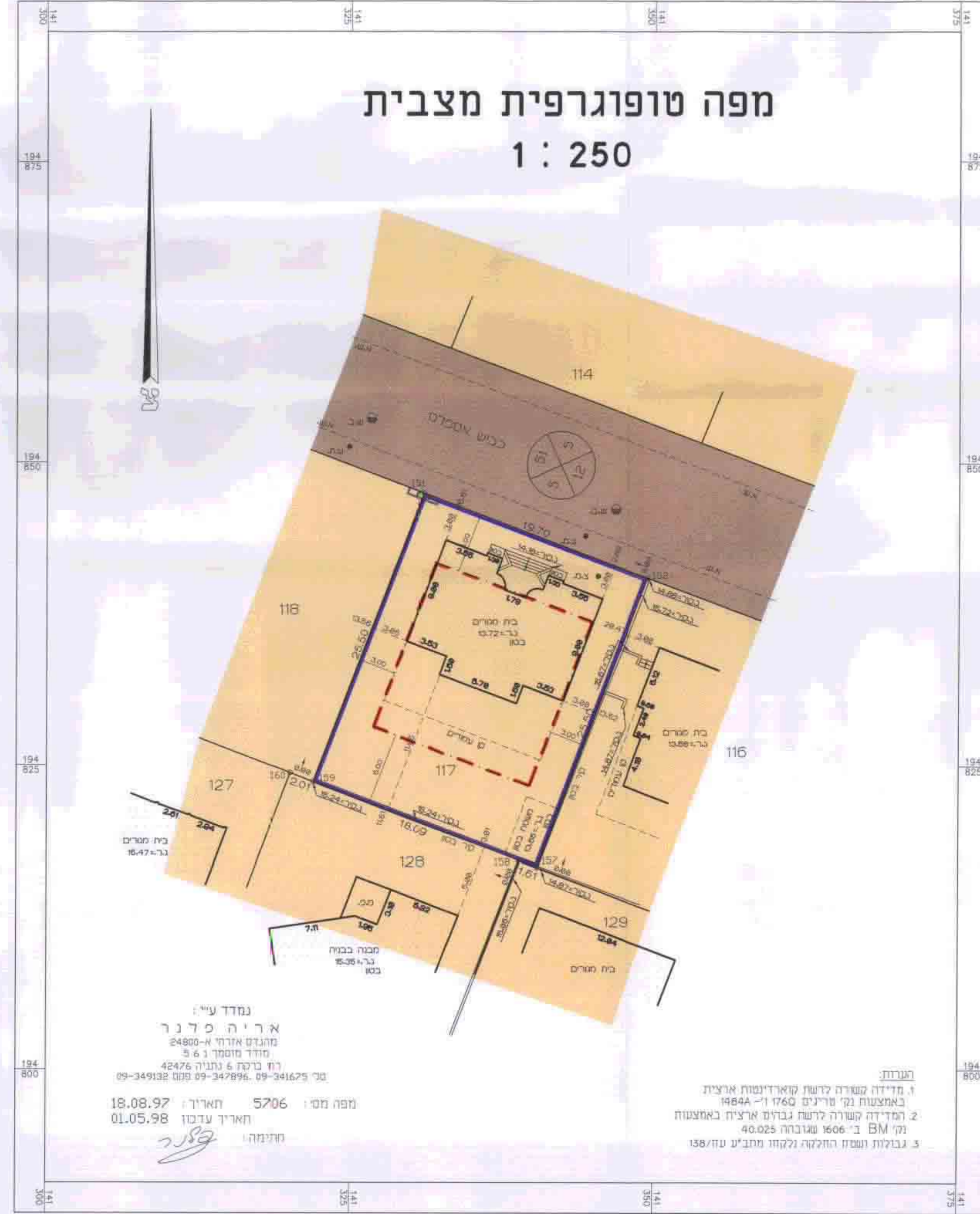
מצב קיים קנימ 1 : 250 לפי עח\במ\163
