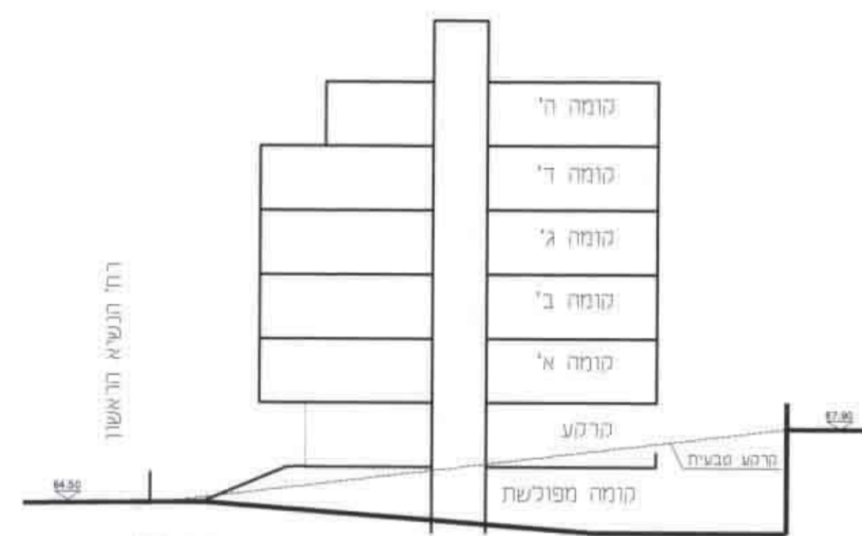
חתך סכמתי לאורך הבנין 1:250
