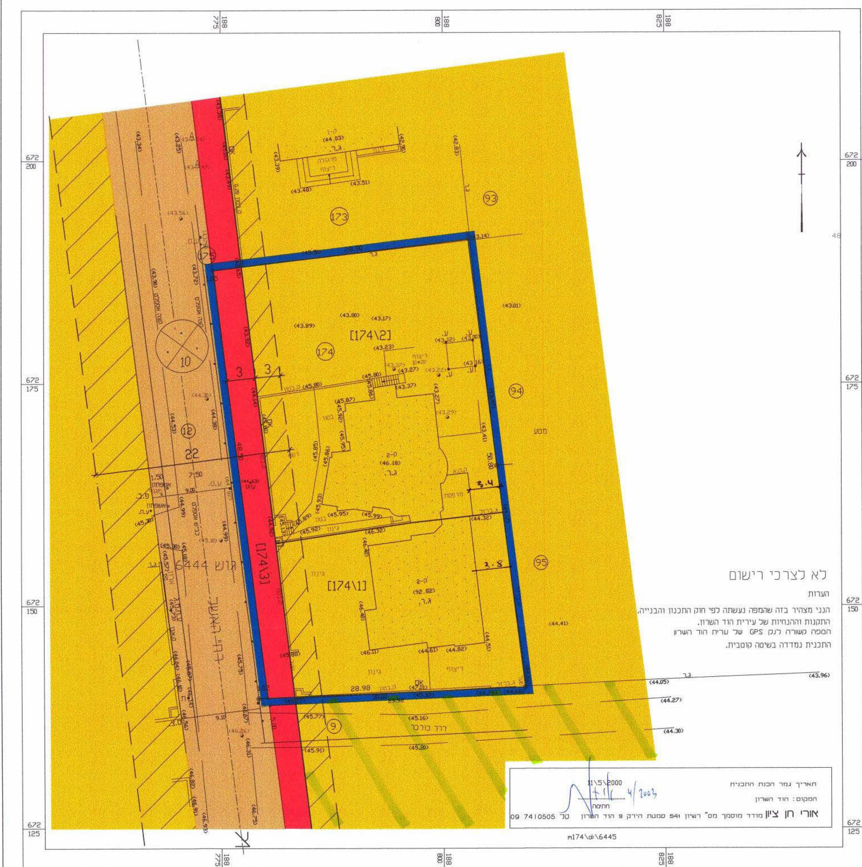
מצב מוצע קרי"מ 1:250
