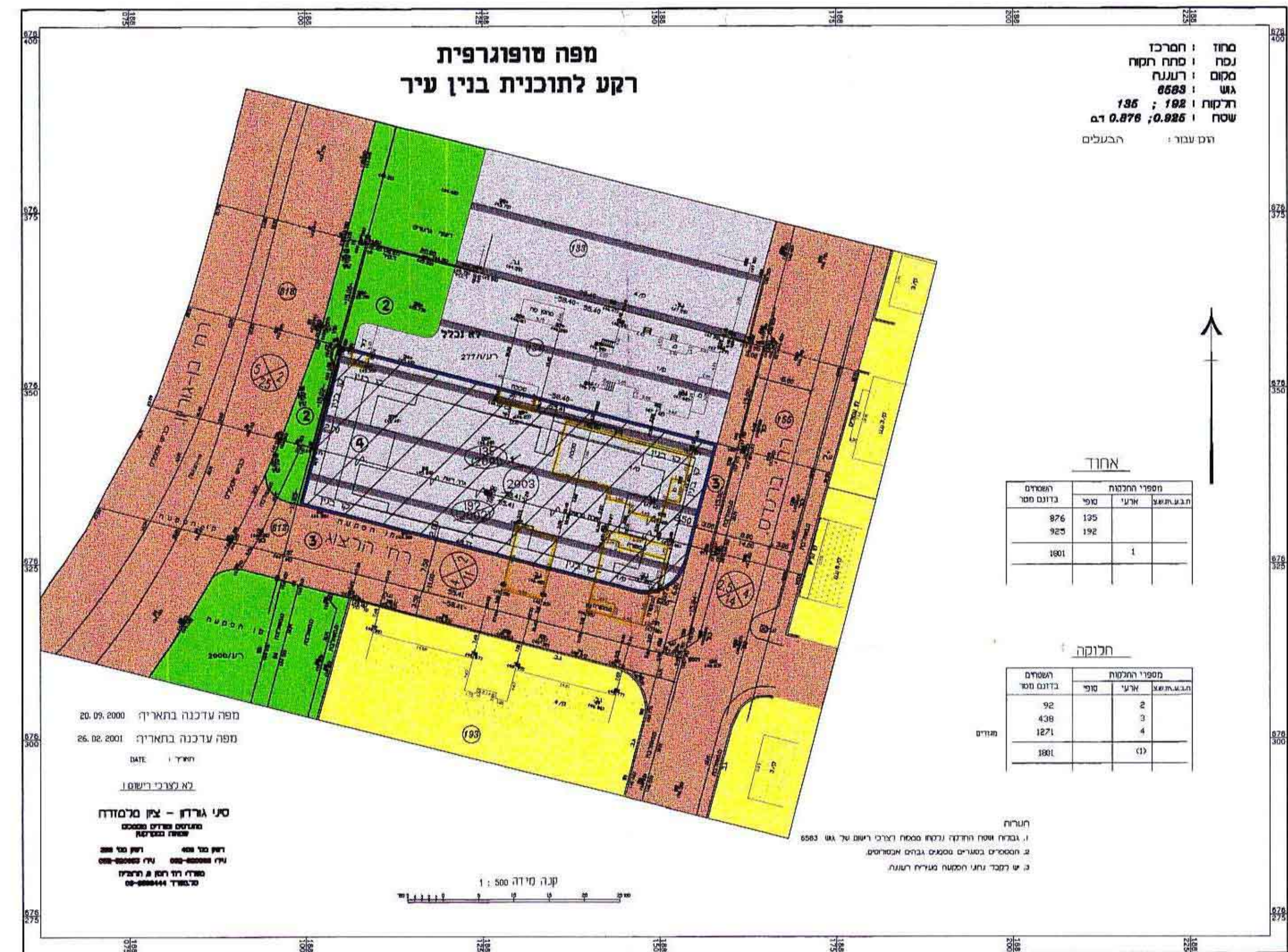
מצב מוצע קני"מ 1:500
