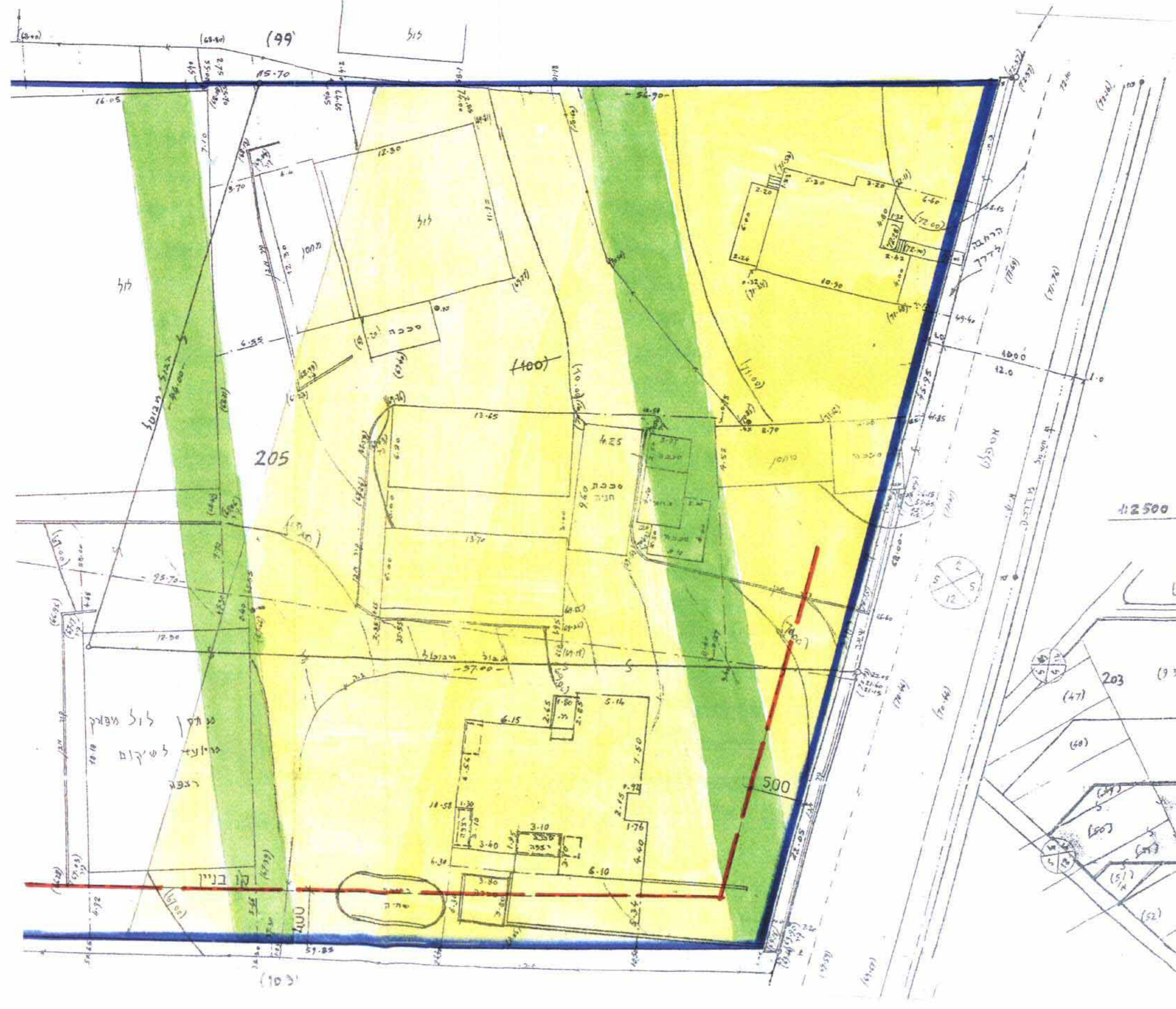
מצב קיים 1:250
