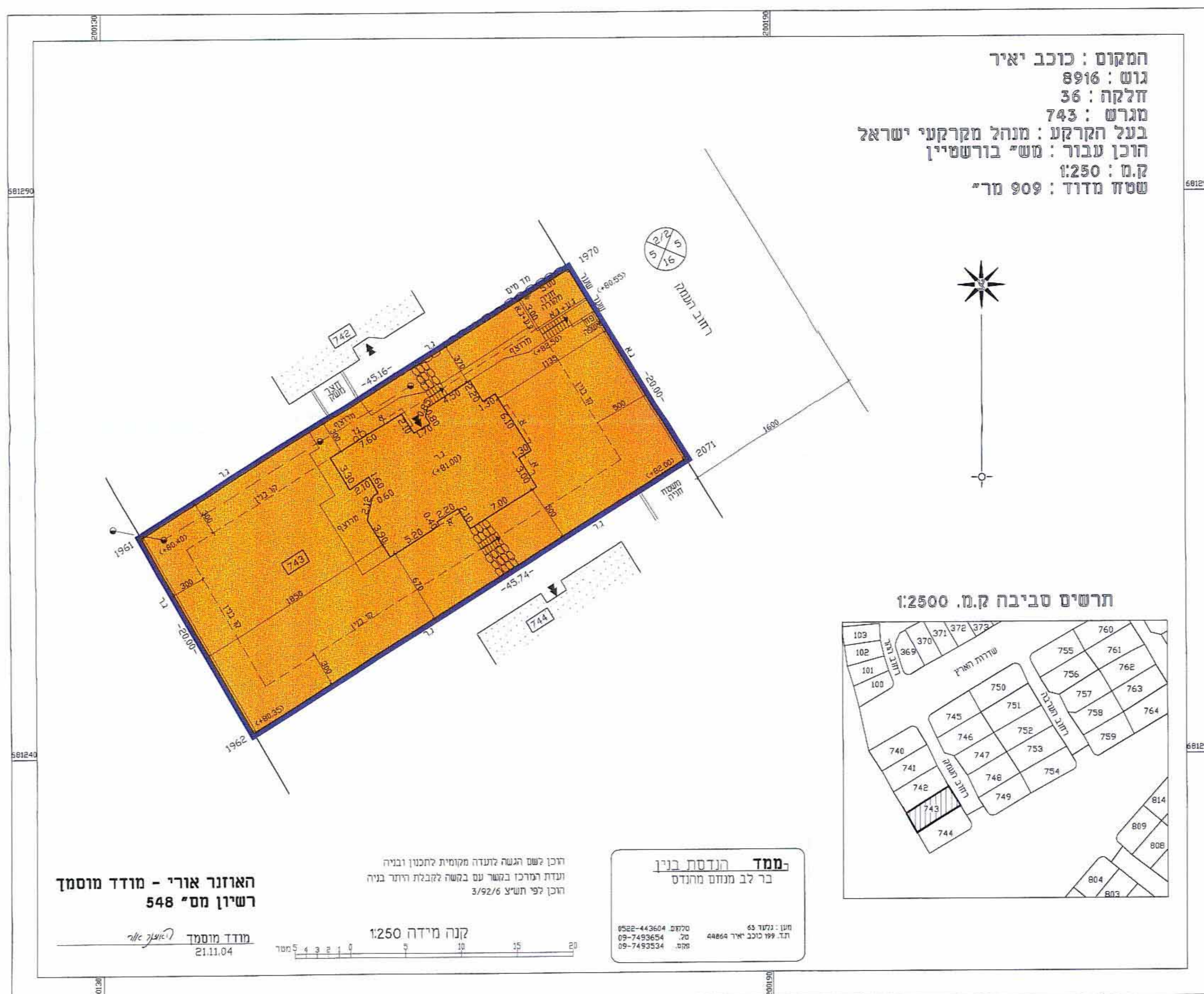
מצב מוצע 1:250
