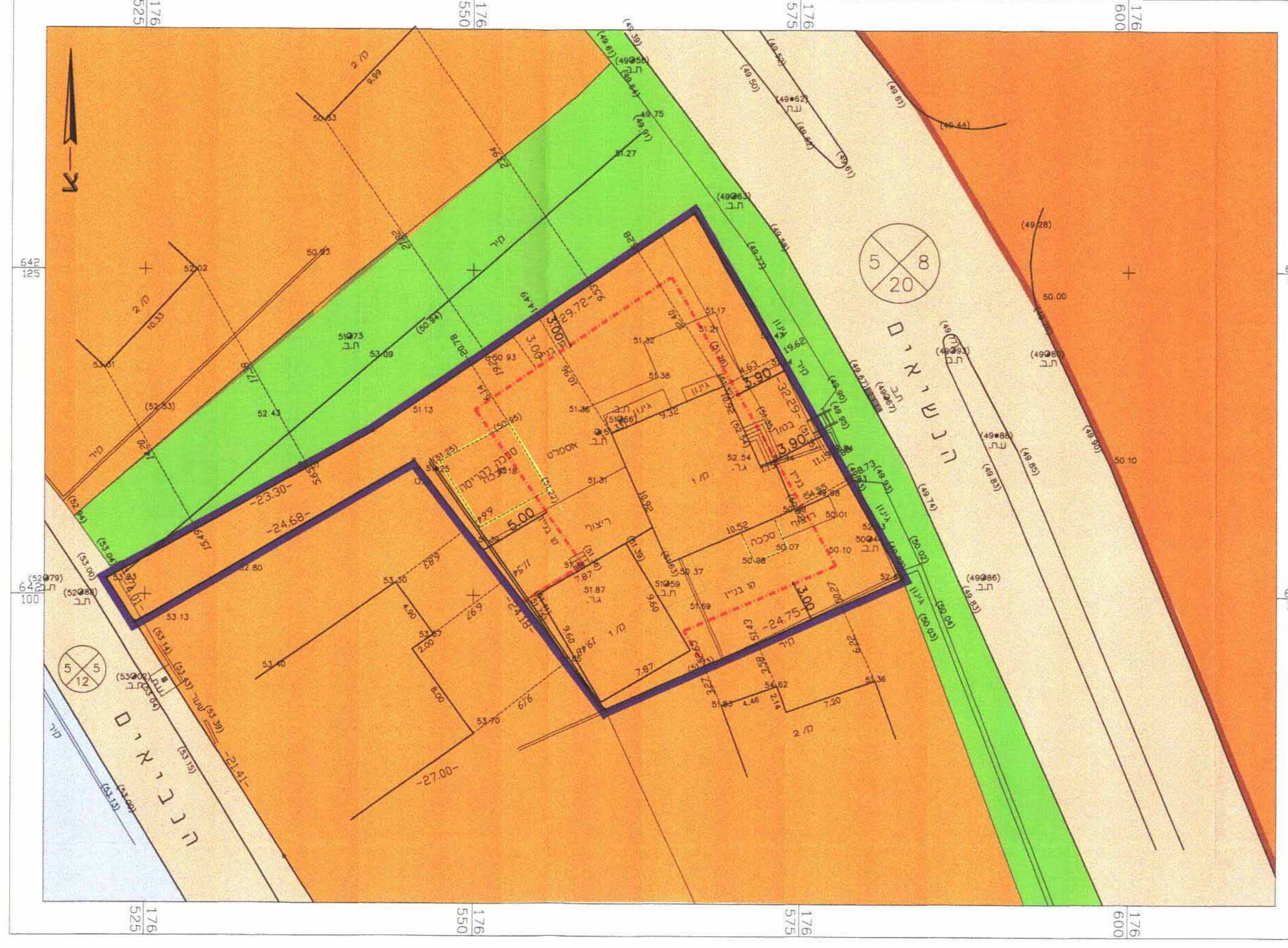
תוכנית מוצעת 1:250
