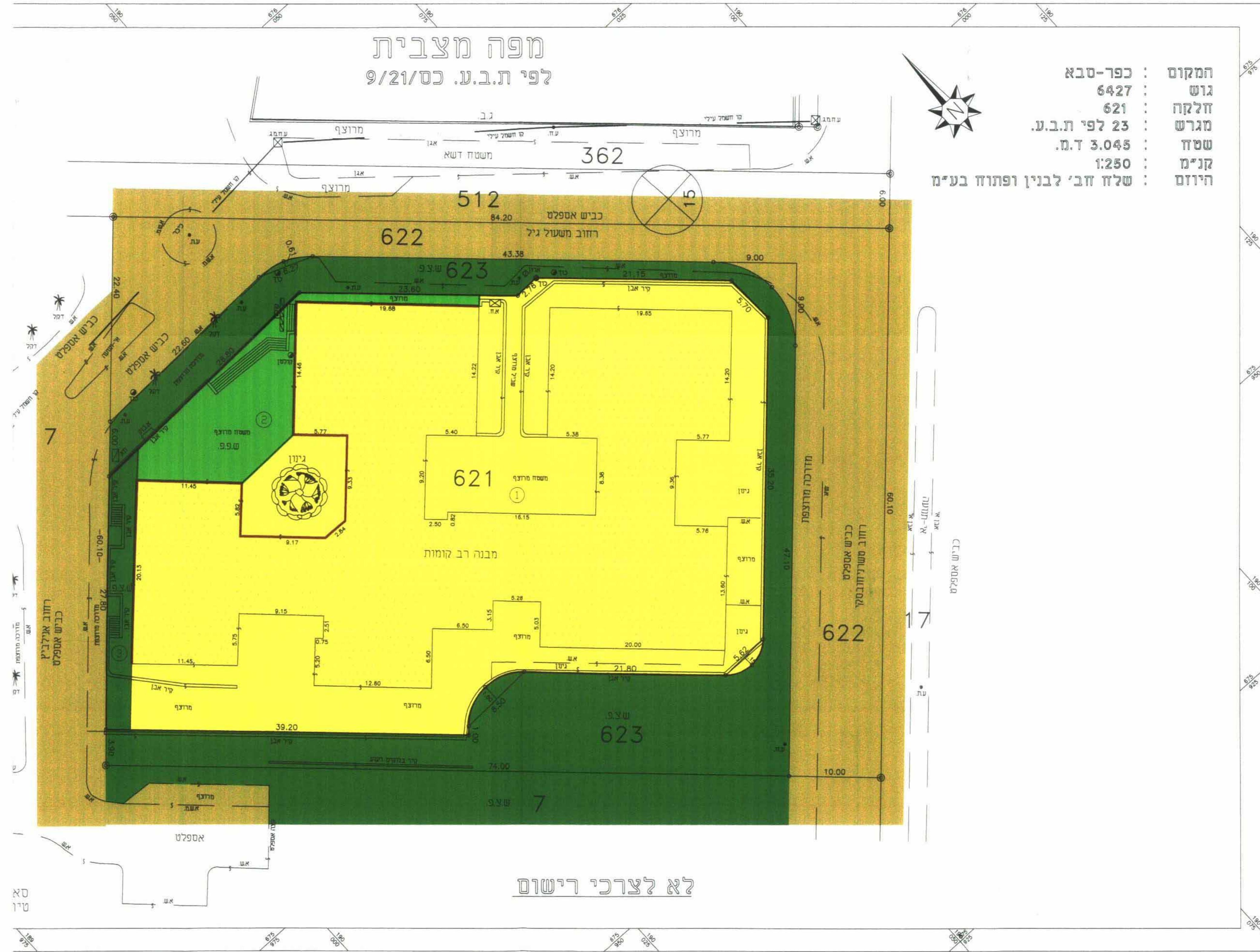
מצב קיים ומוצע 1:250
