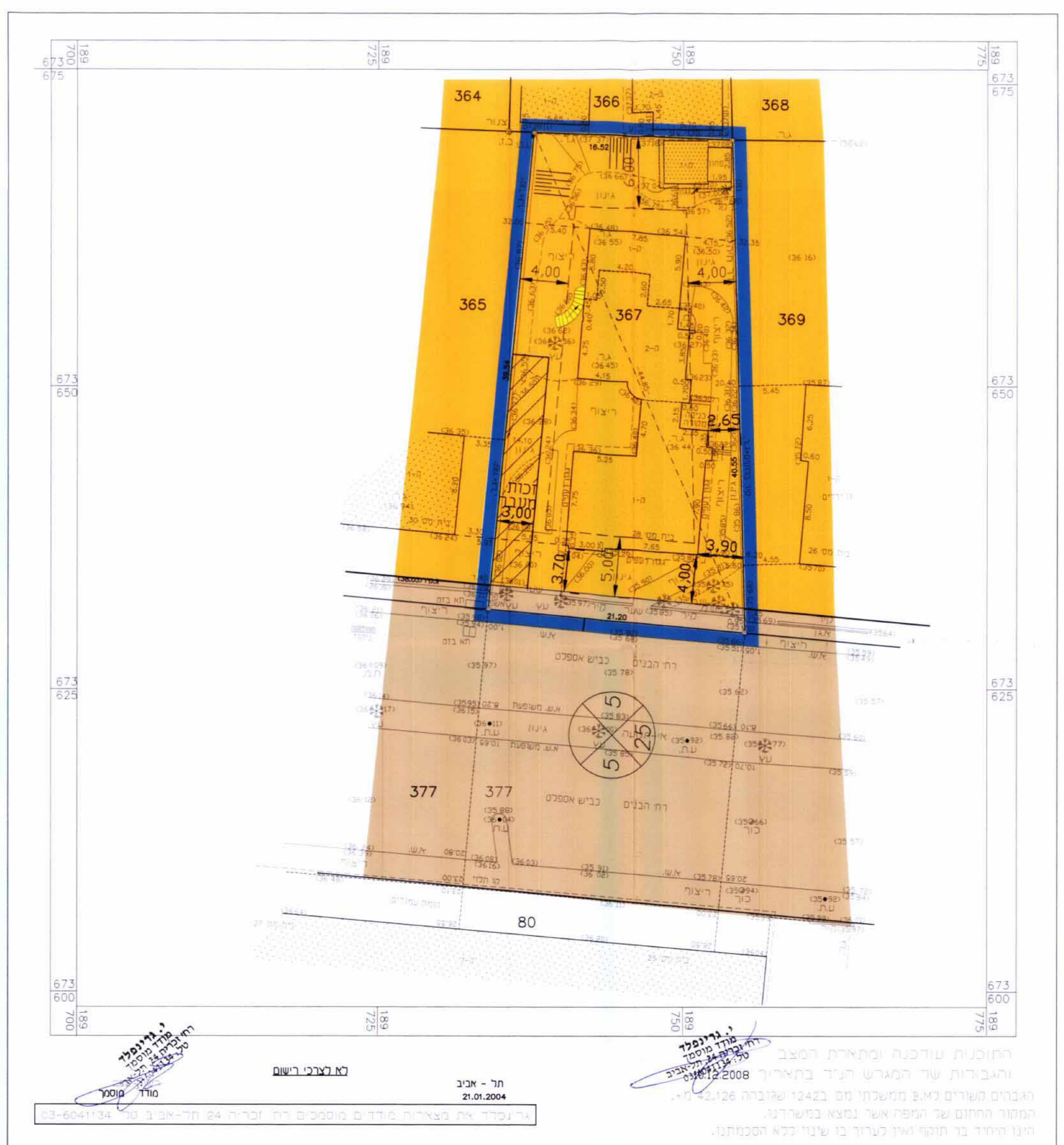
מצב מוצע קני'מ 1:250
