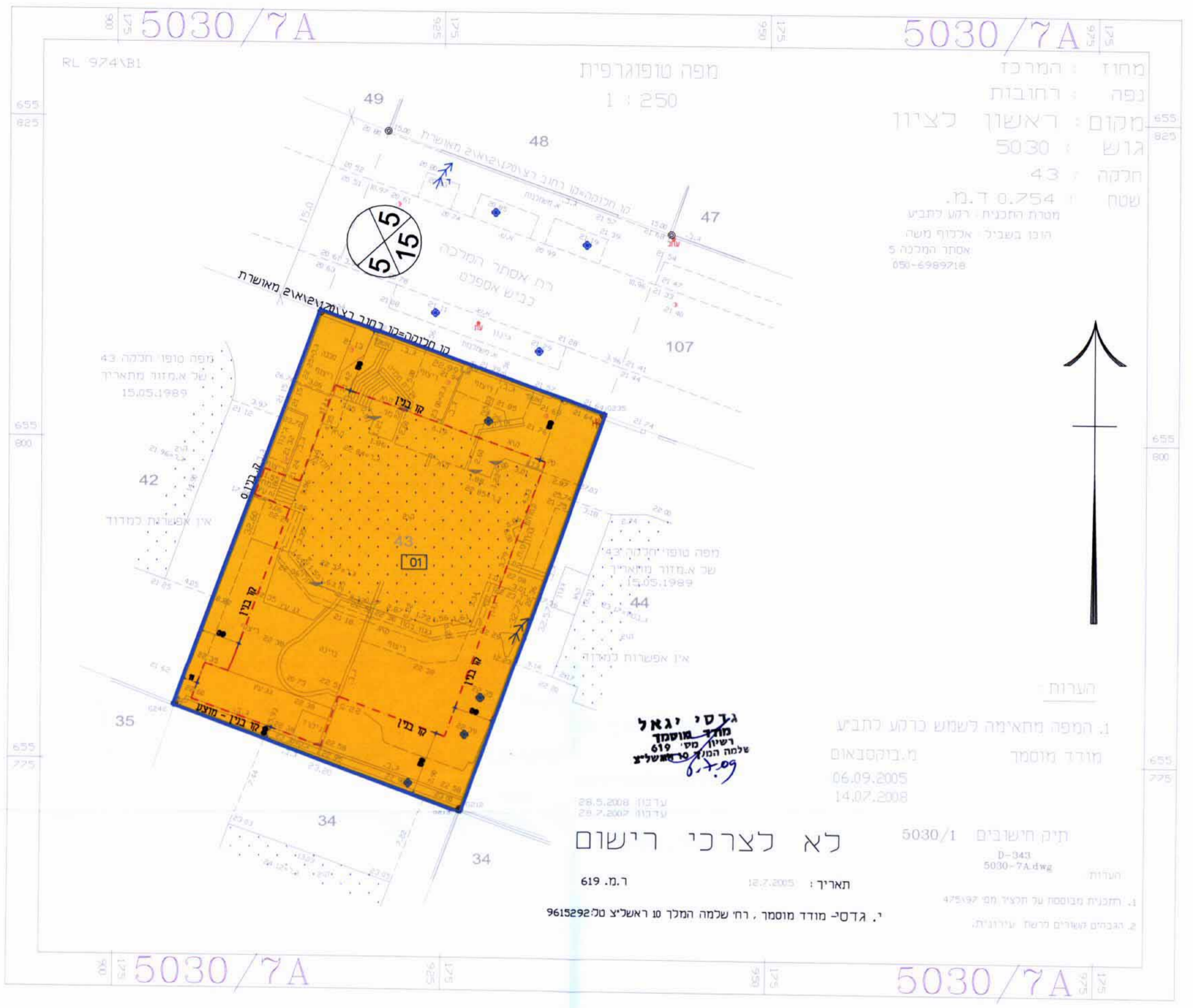
מצב מוצע קנ"מ 1: 250
