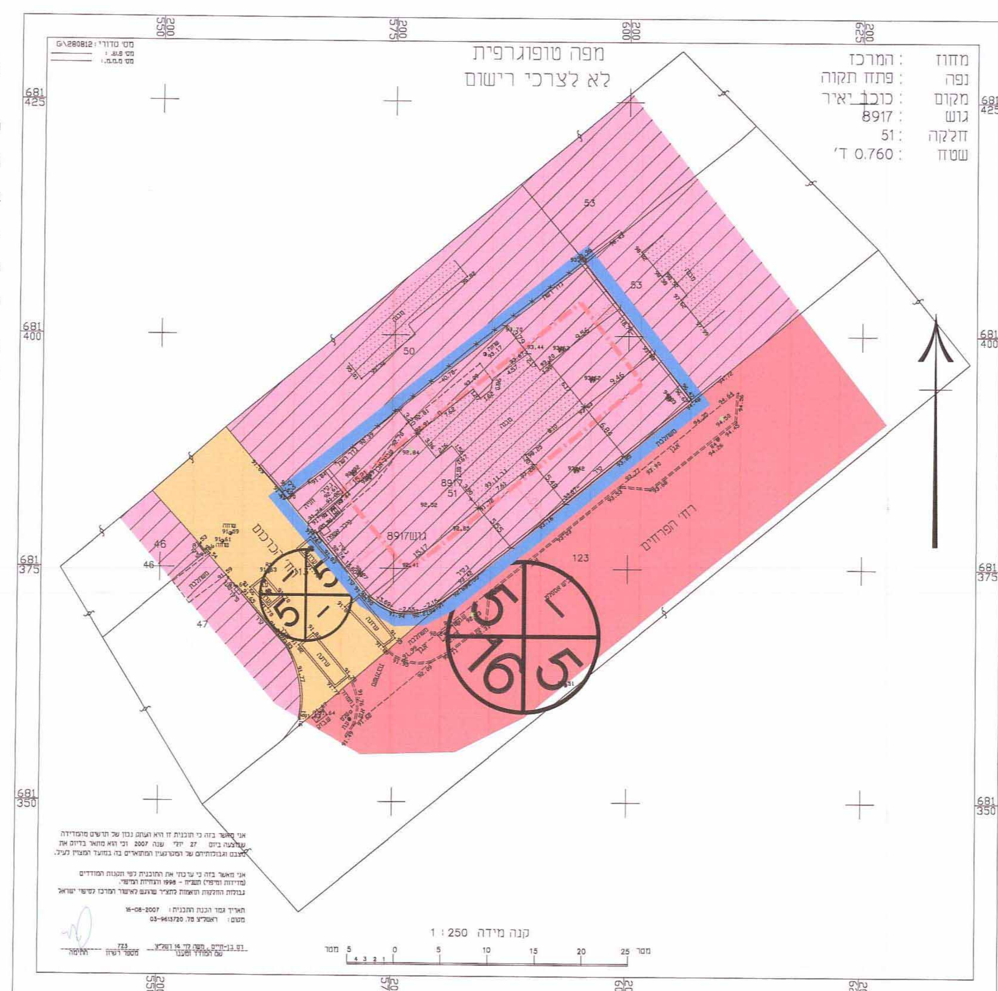
מצב מאושר קני"מ 1: 250
