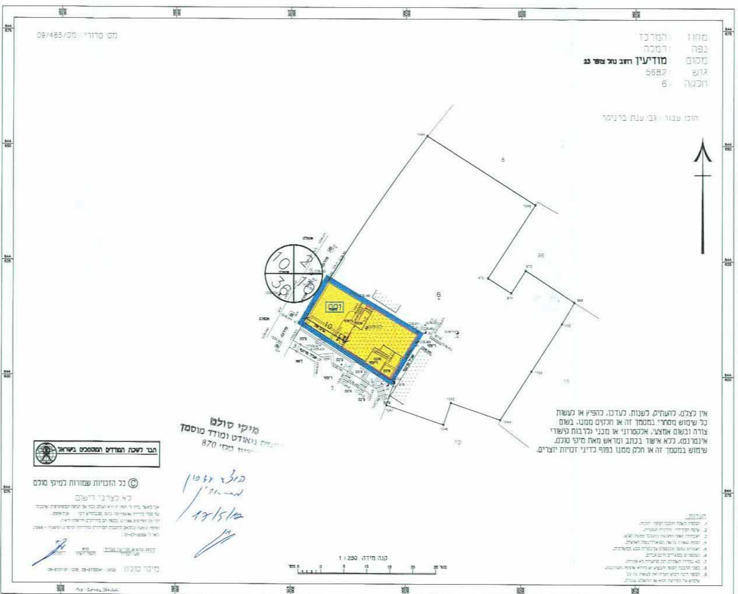
מצב מוצע קנ"מ 1:500
