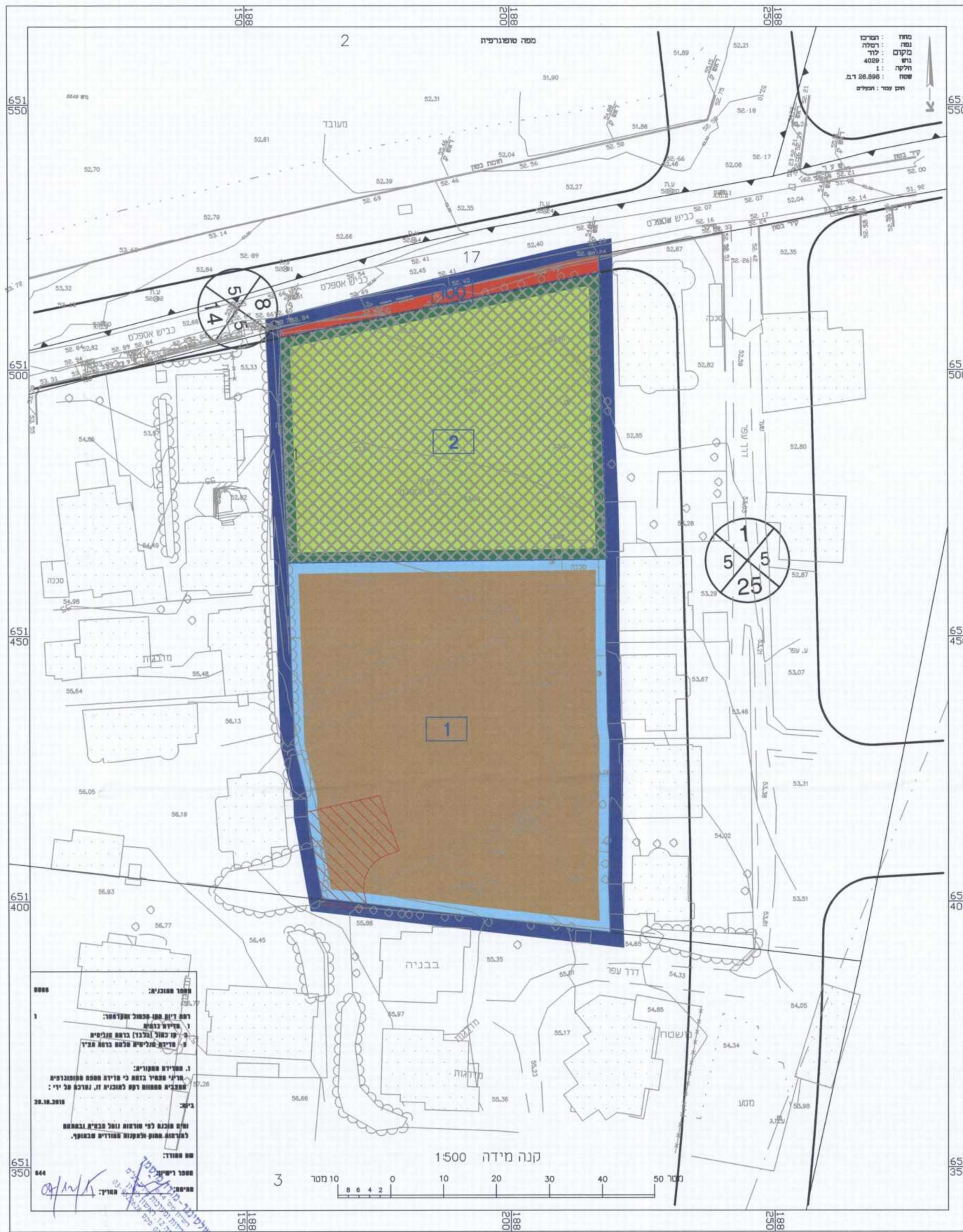
מצב מוצע קנ"מ 1:500
