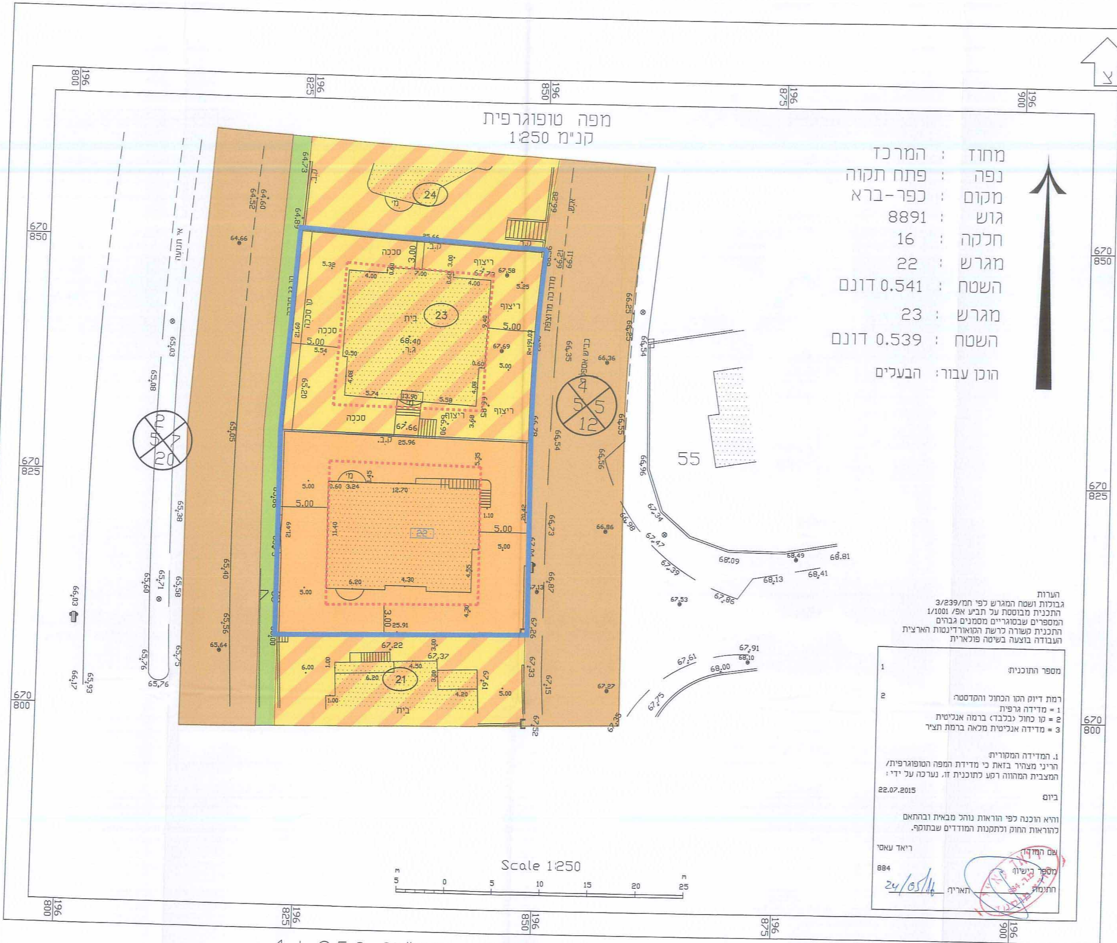
מצב מאושר קנ"מ 1 : 250 לפי תכנית ק/1001 לפי תכנית ק/מק/3566
