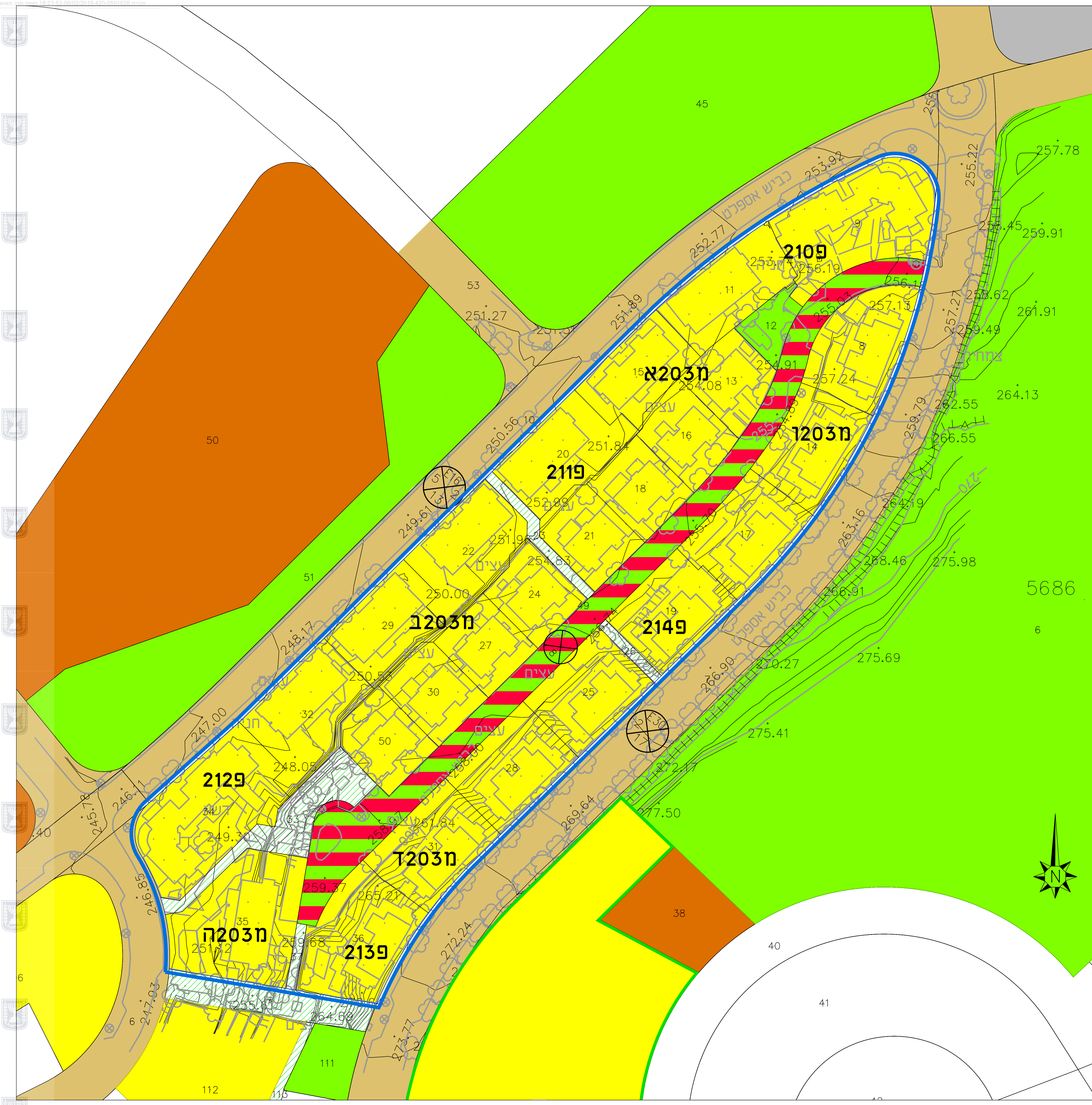
מצב קיים 1:500
