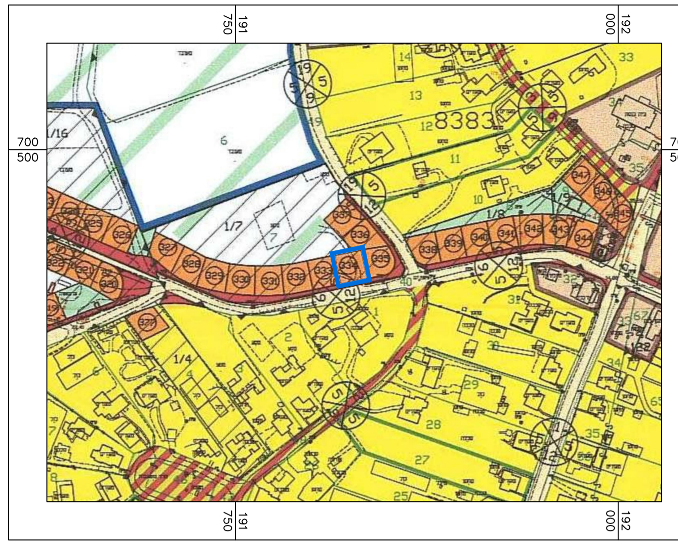
תרשים הסביבה לפי עח\143\8 קנ"מ 1:2500
