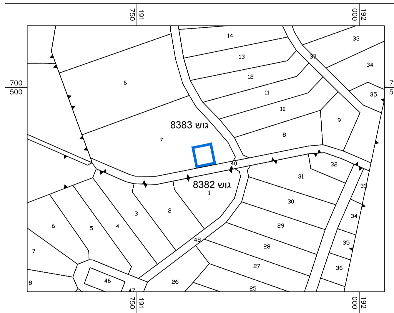
קנ"מ 1:2500 גושים חלקות
