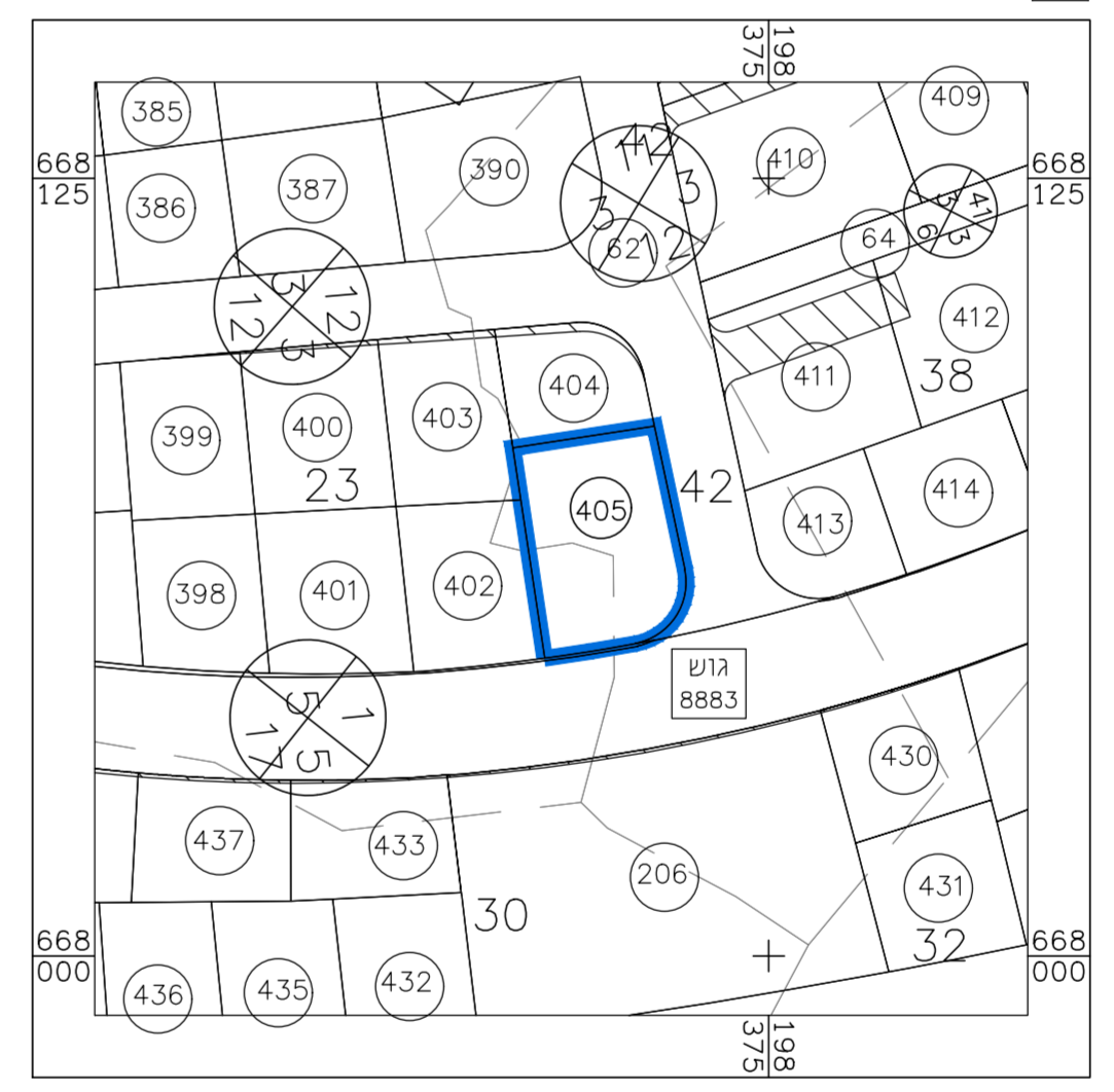
תרשים לטביבה הקרובה קנ"מ 1 : 1250
