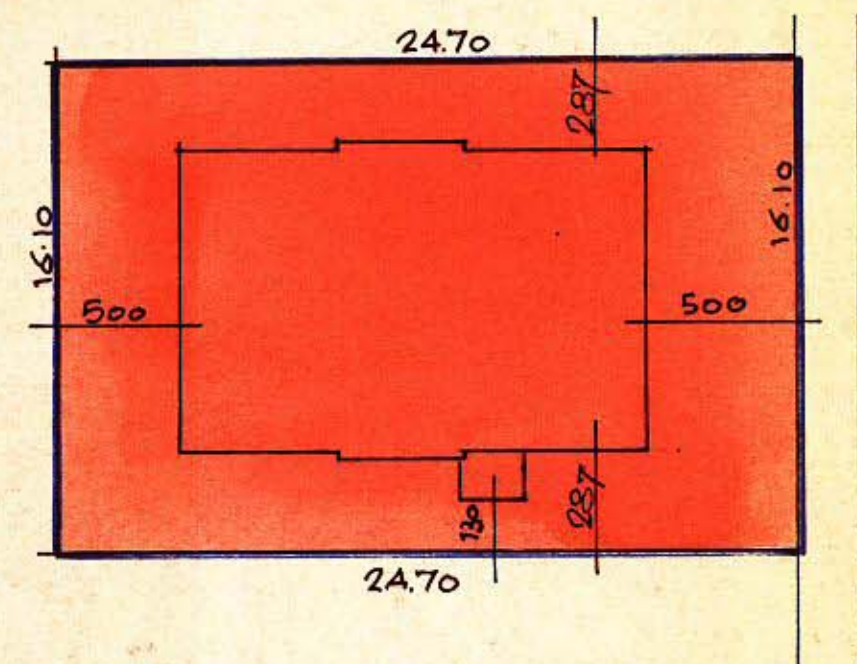
מטב מוצע 1:250
