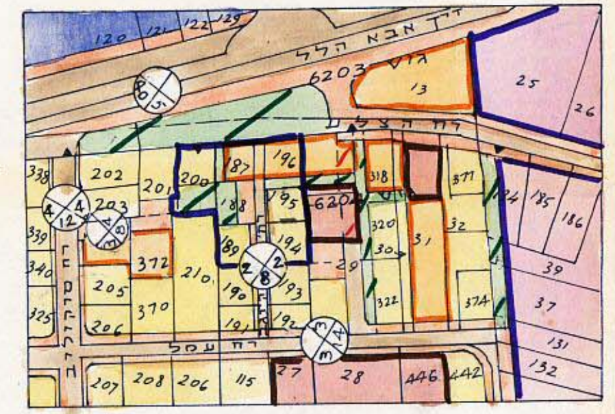
מצב קיים לפי תכנית מפורטת רג/204 DE ק.ל. 1:2500
