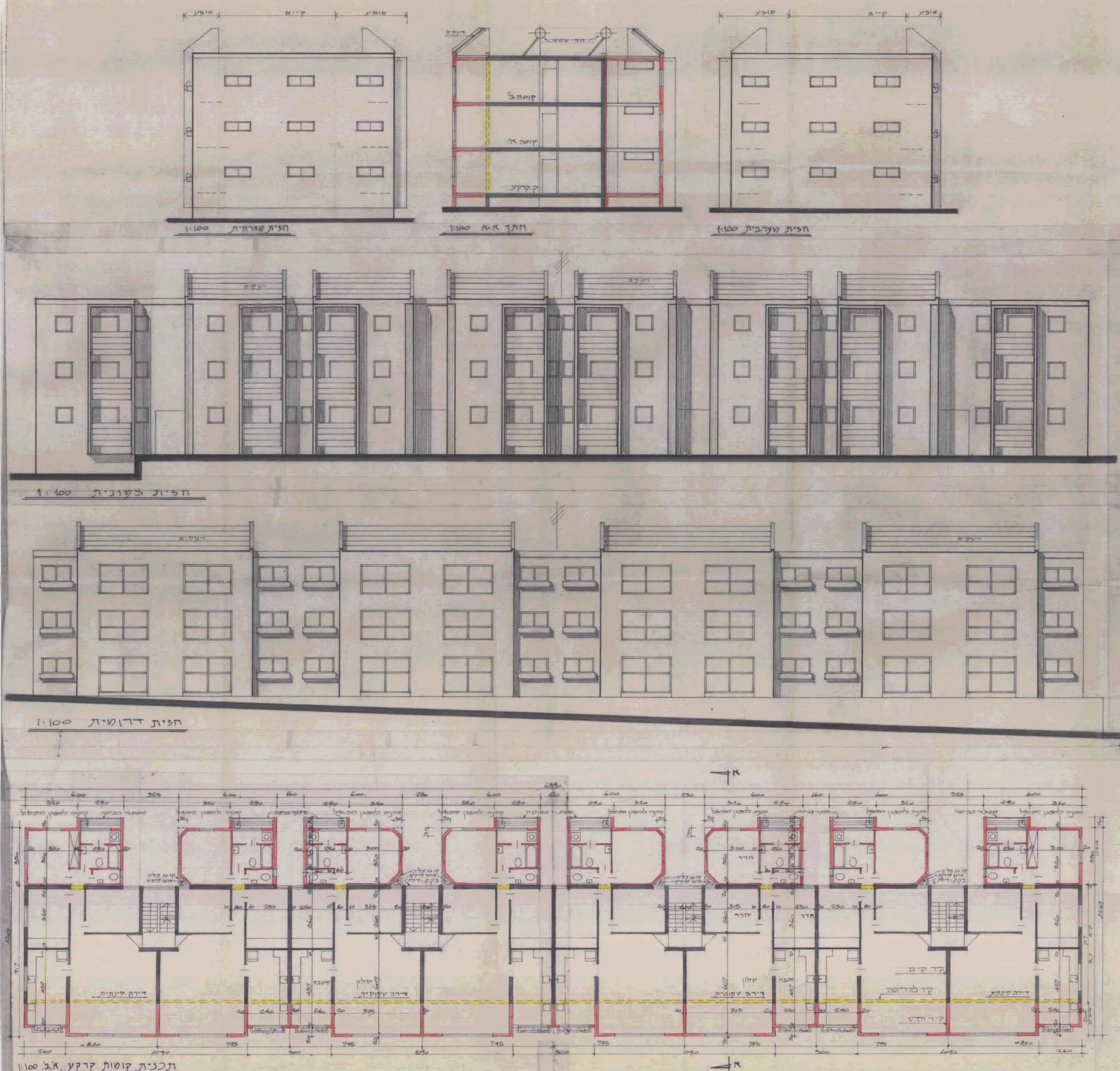
תכנית קומות קרקע, א.ב. 1:100
