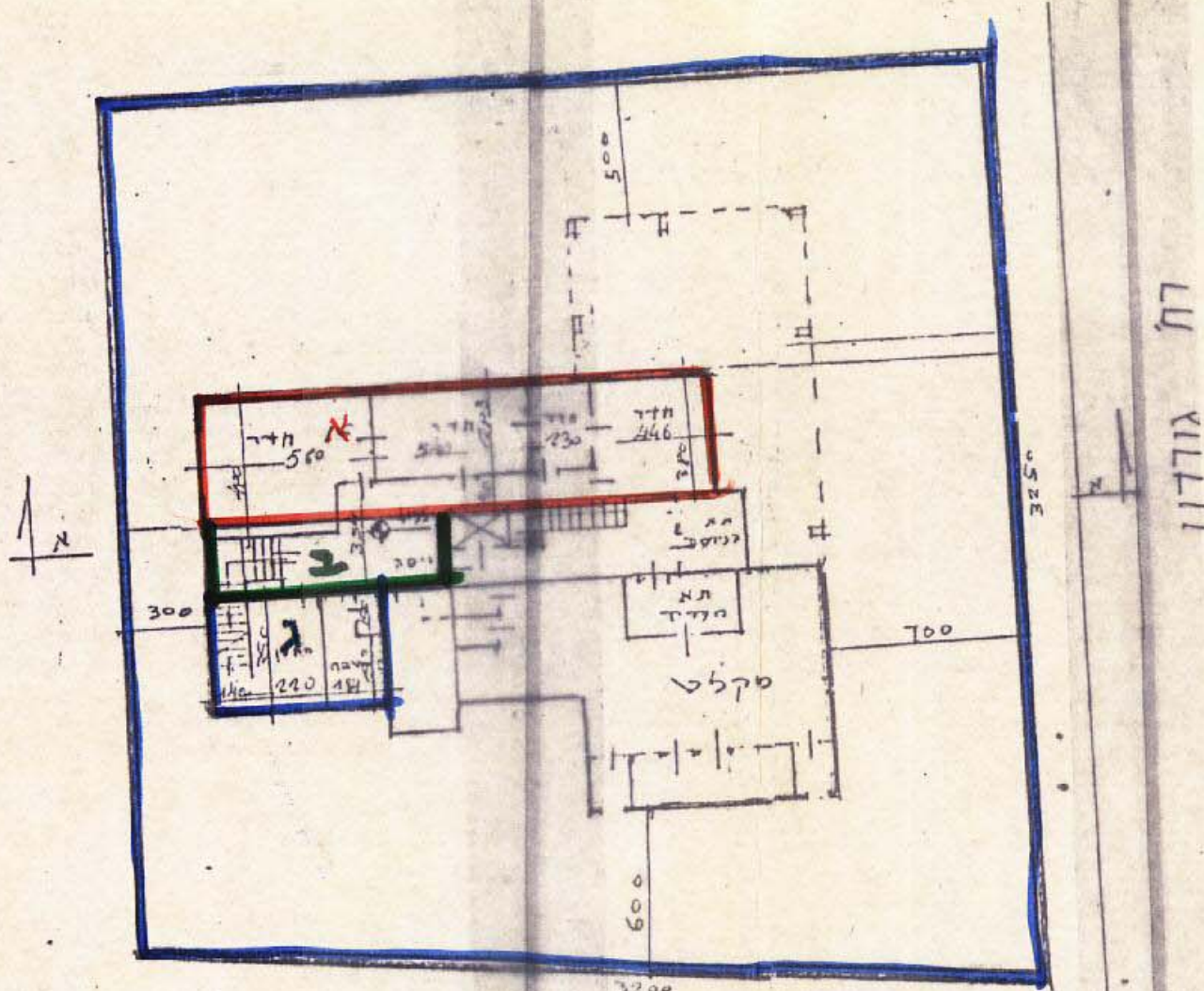
תכנית קומת מרתף מוצע ק.מ. 1:250
