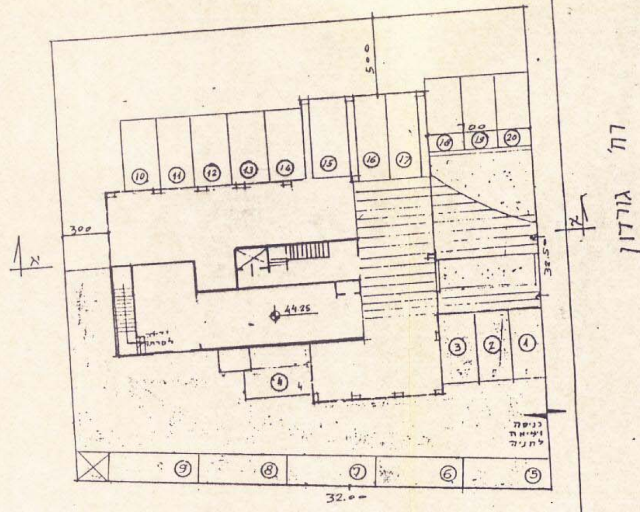
תכנית קומת הקרקע מוצע ק.מ. 1:250
