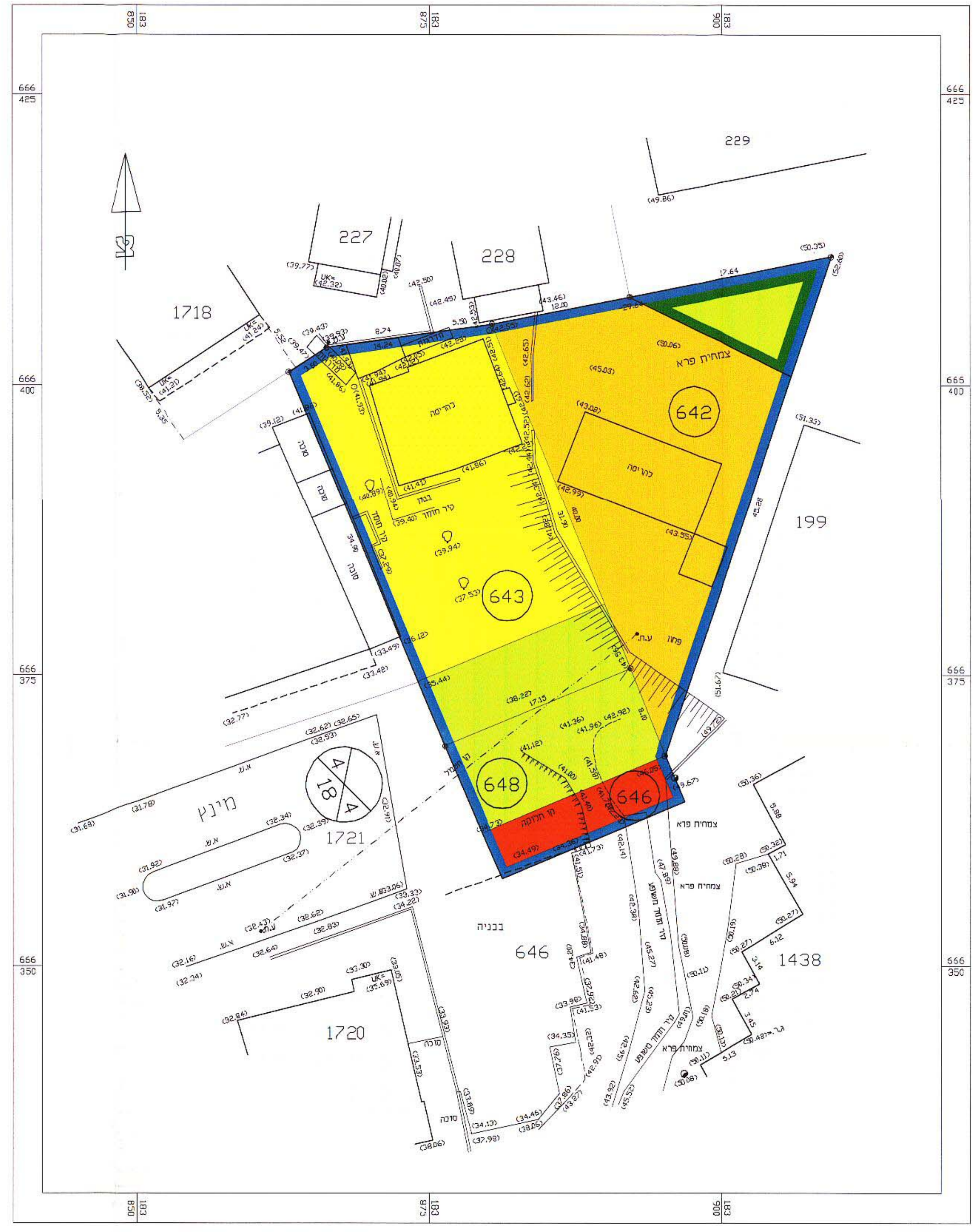
תרשים מוגרש קני"מ 1:250 מצב קיים
