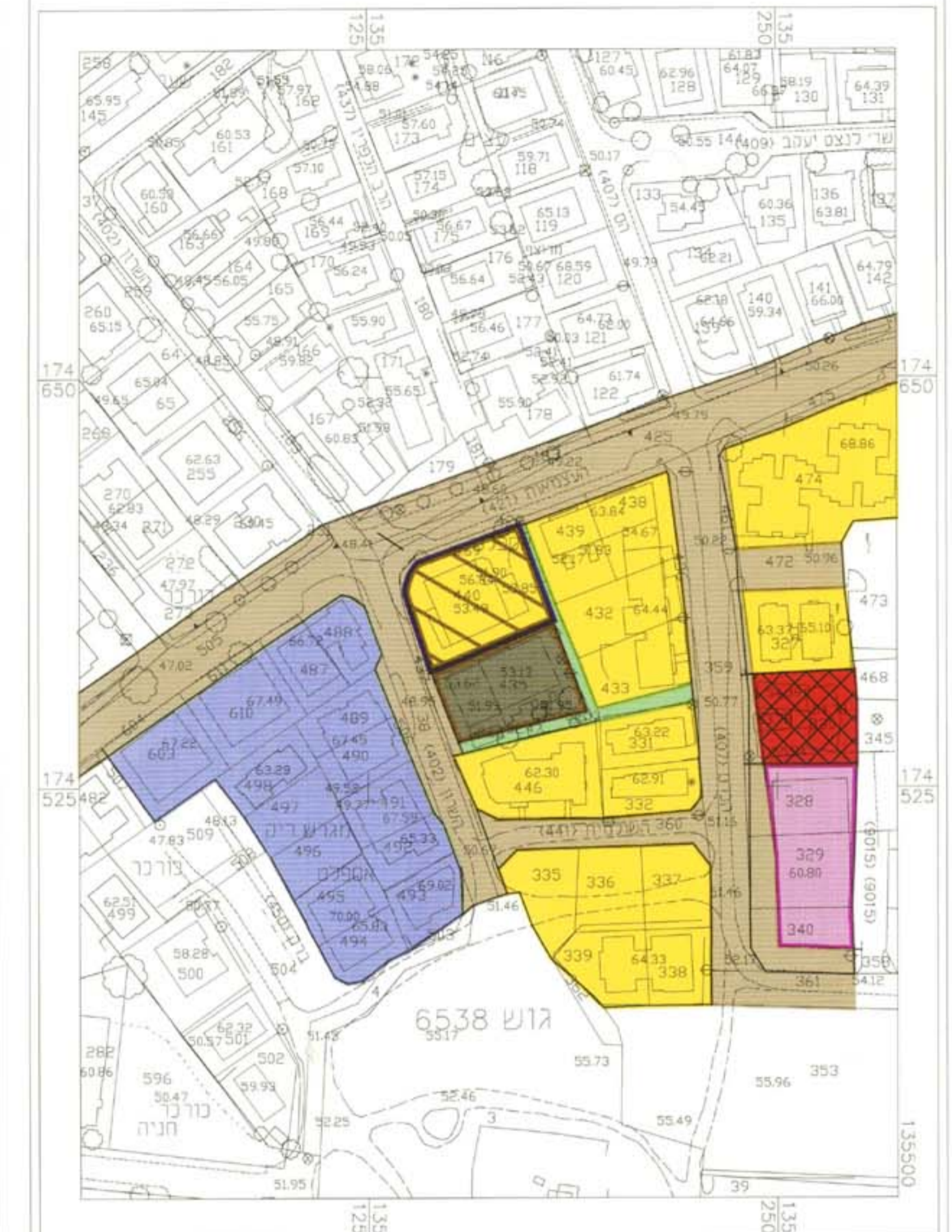
תכנית שביבה מצב קיים ע"פ תכניות מס' הר/1316, הר/570, הר/447, הר/1089 ק.מ. 1:1250
