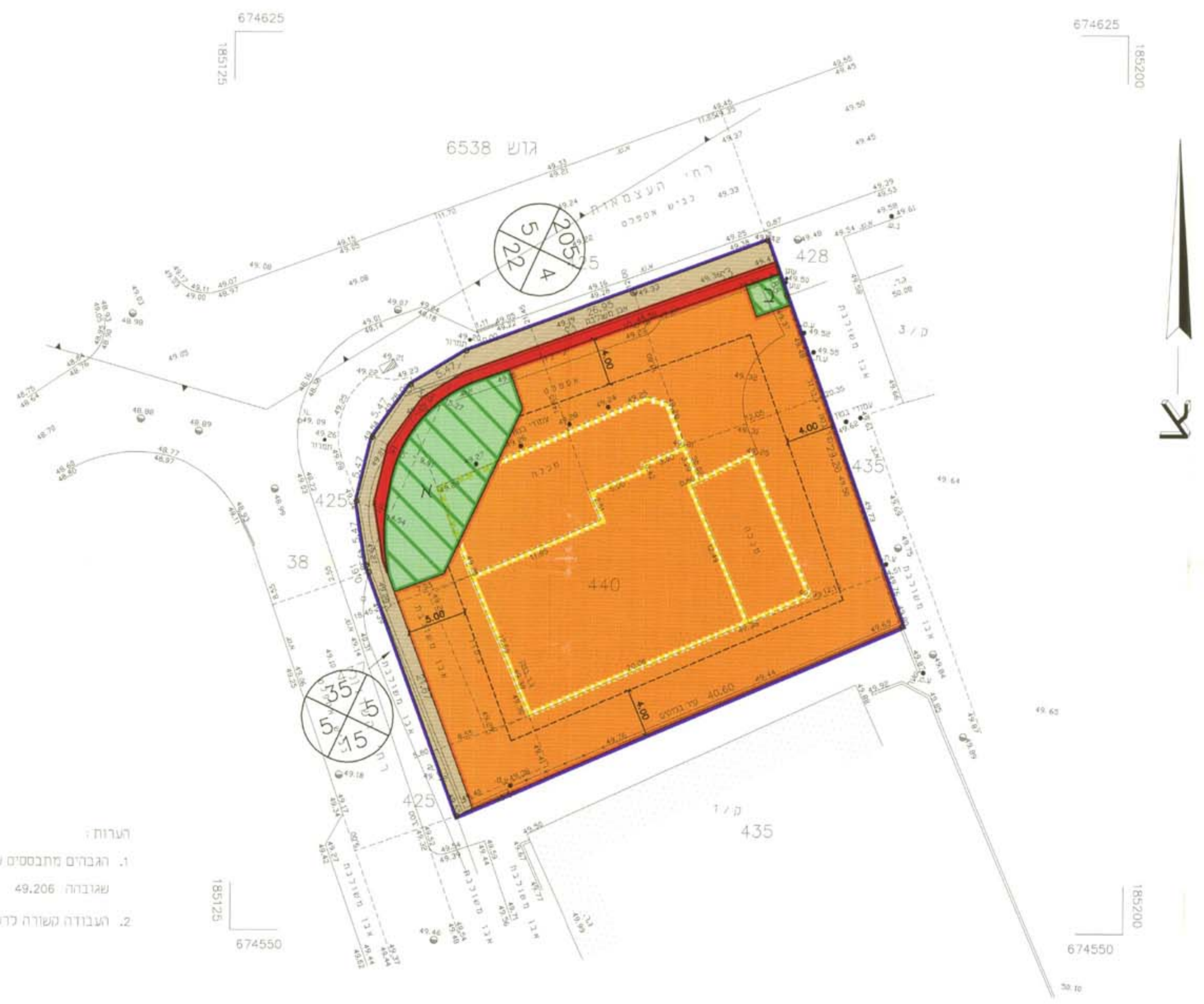
מצב מוצע ק.מ. 1:250
