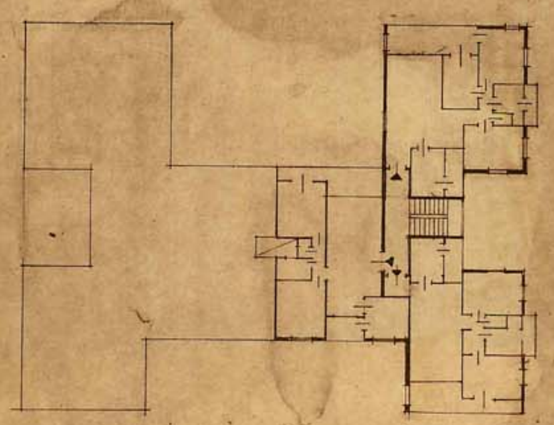
תכנית קומה טיפוסית ק.פ. 1:200
