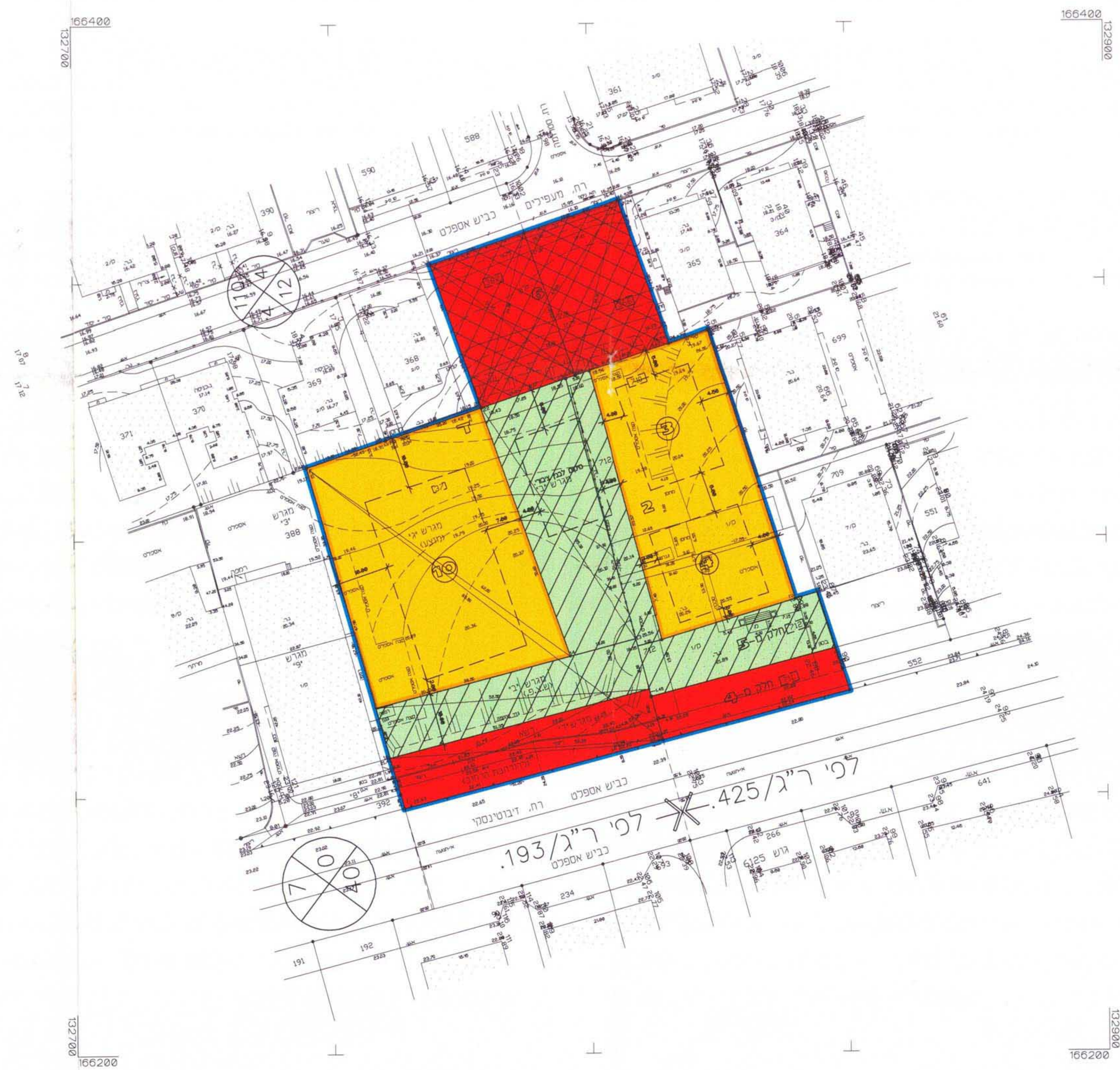
מצב קיים ק.מ. 1:500
