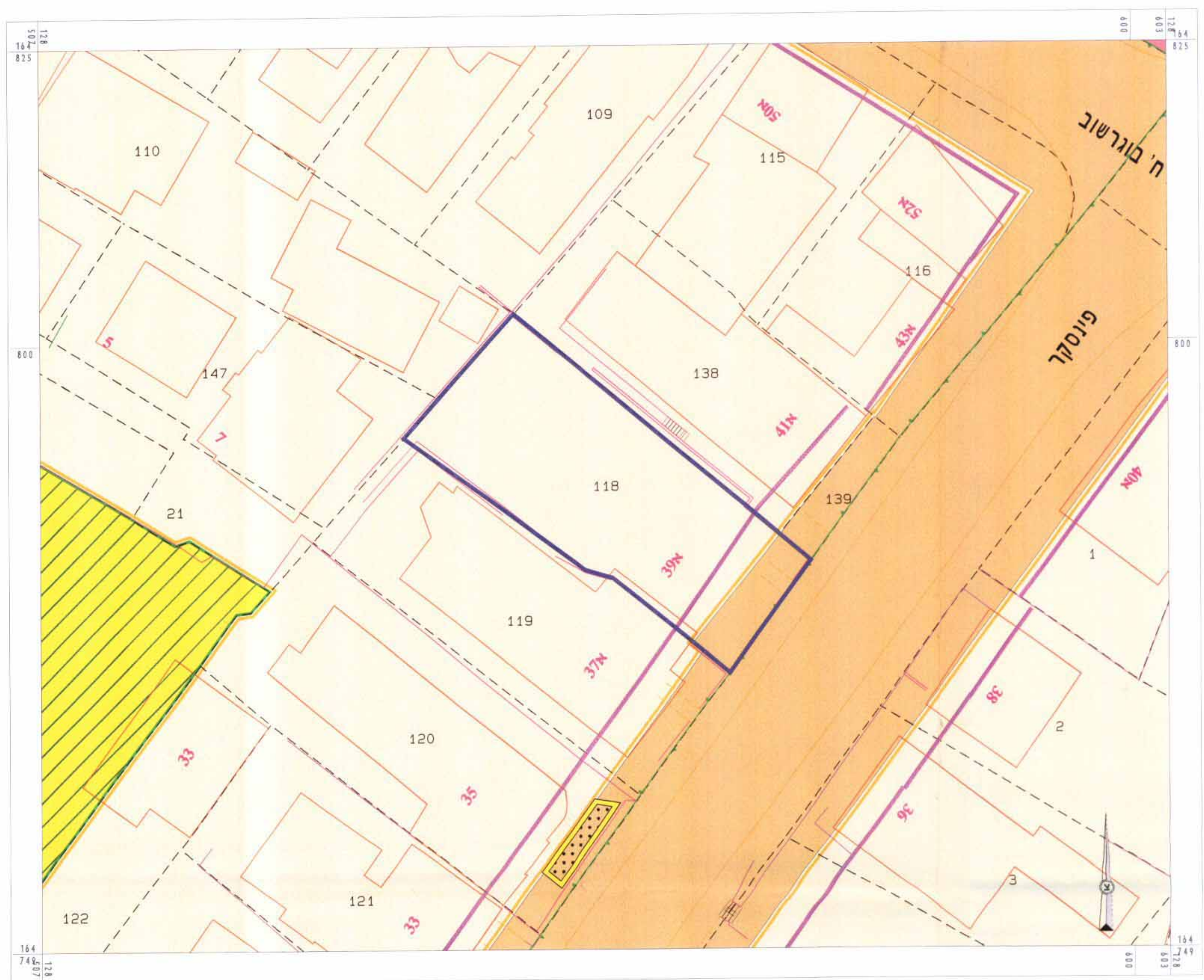
תכנית מצב קיים קנ"מ 1:250
