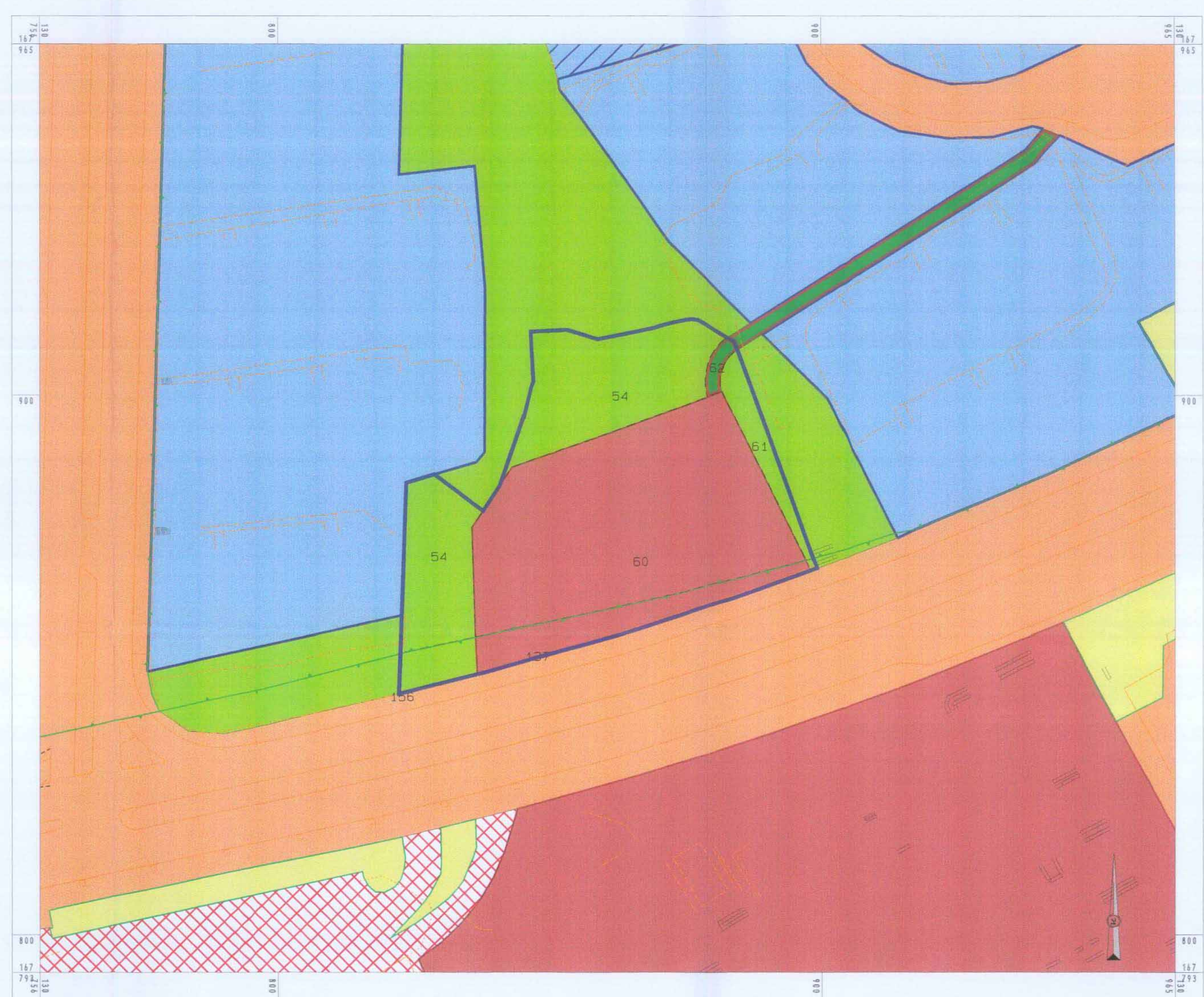
תכנית מצב קיים קנ"מ 1:500
